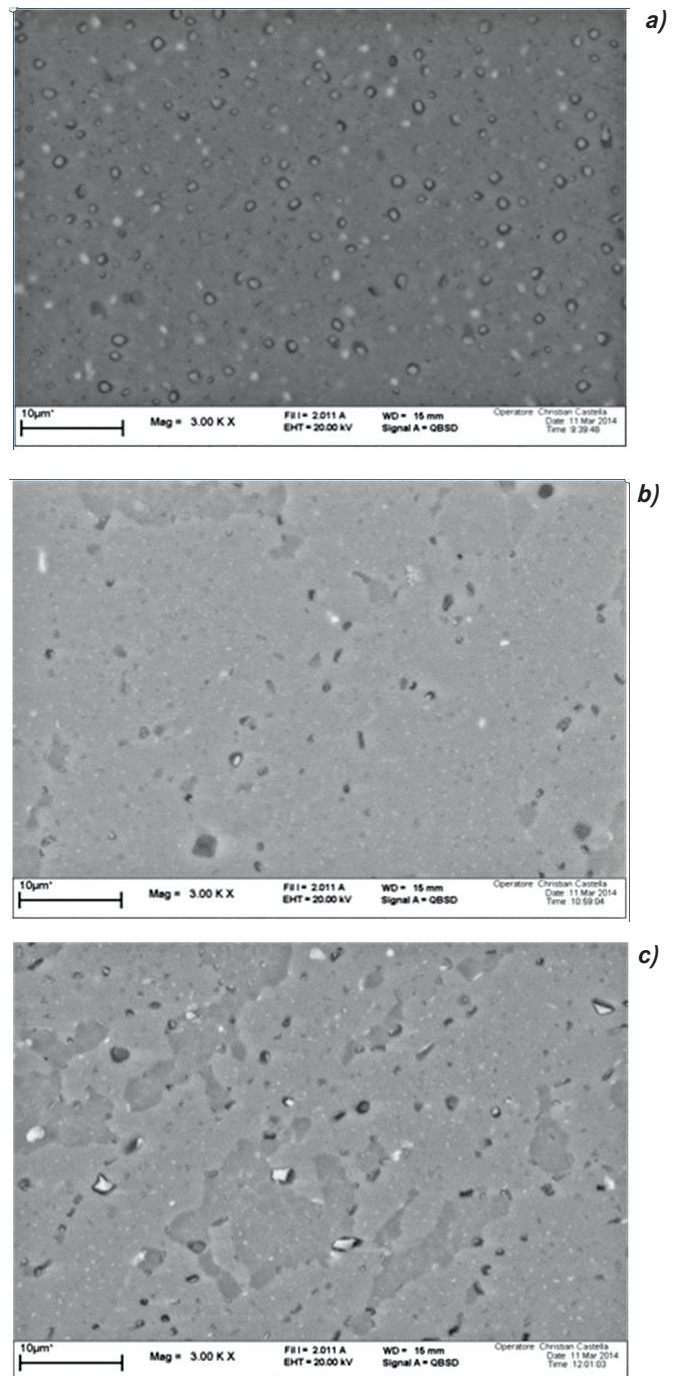
Fig. 3 - Micrografie SEM dei campioni: a) campione serie 1; b) campione serie 2 e c) campione serie 3.
