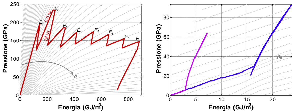
Fig. 9: Percorso (ottenuto dalla simulazione a fronte della definizione di EOS polinomiali) sulla EOS tabulare originale (linee sottili chiare) per l'elemento in cui è stato depositato il livello massimo di energia (sinistra), per un elemento esterno alla zona di massima deposizione (destra, blu) e per un elemento sulla superficie esterna (destra, magenta)
