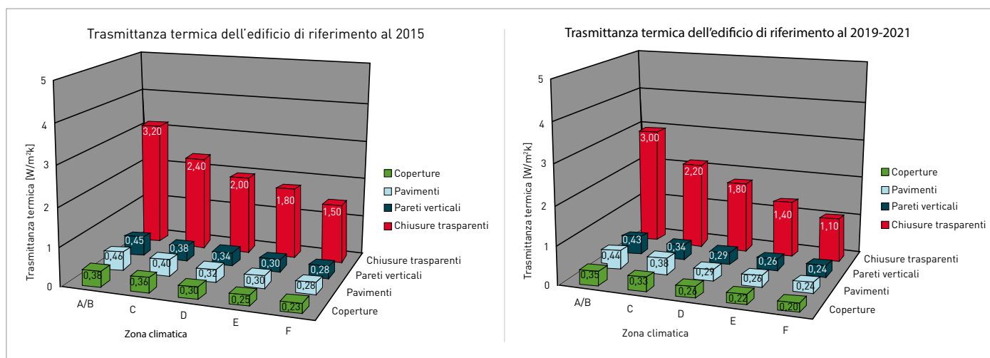
Figura 5: Valori di trasmittanza termica dell'edificio di riferimento.
