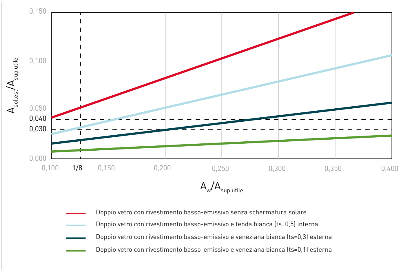
Figura 14: Correlazione tra A_{sol,est}/A_{sup,utile} e A_{w,p}/A_{sup,utile}
