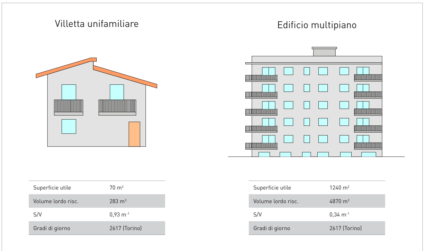
Figura 12: Casi studio analizzati per rappresentare la tendenza storica dell'isolamento termico dell'involucro.
