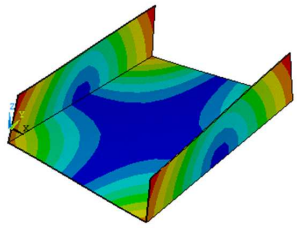
(a) Config. Fig. 4 (a) Mode 1: ANSYS
