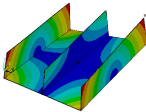
(b) Config. Fig. 4 (b) Mode 1: ANSYS
