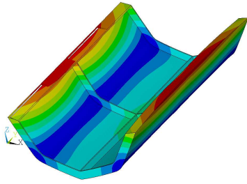
(c) Mode-2: ANSYS
