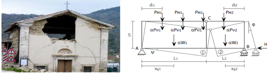
Figura 5. Estrutura atingida por mecanismo de flexão horizontal de parede e modelo cinemático.
