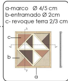
panel en bambú con revoque en tierra
