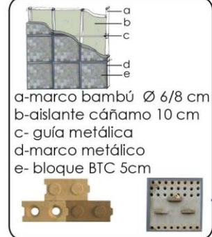
revestimiento paneles tierra y aislante cáñamo
