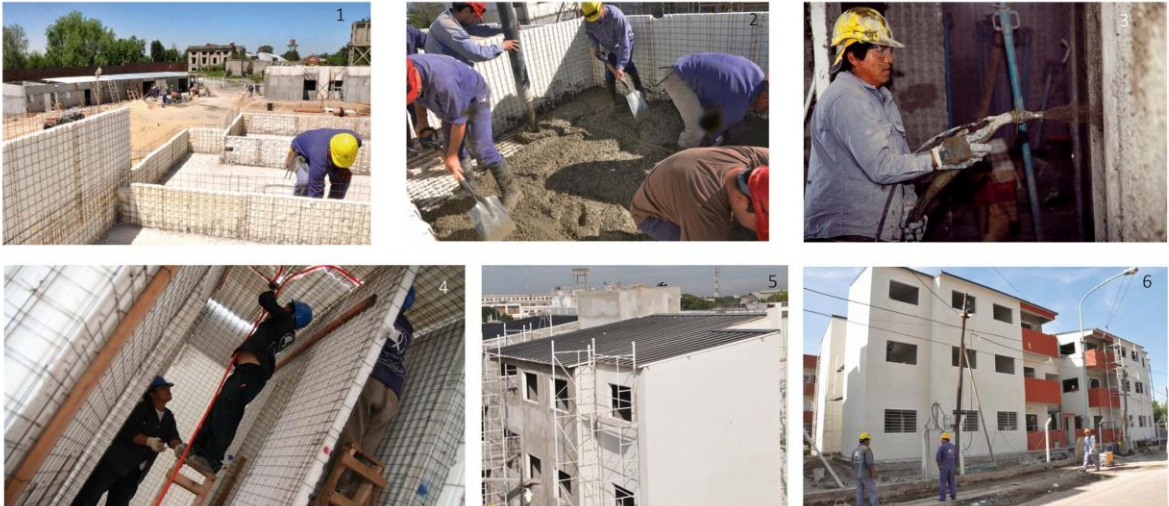
Fotos 1 a 4: montaje de los paneles, llenado con cemento proyectado y pases de instalaciones. Foto 5 y 6: cubierta inclinada y vista general de uno de los edificios. fuente: www.facebook.com/pages/Misión-Sueños-Compartido
