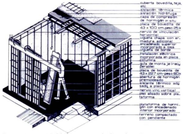
Componentes y montaje del sistema estructural y de envoltura BENO. Fuente: www.ceve.org.ar
