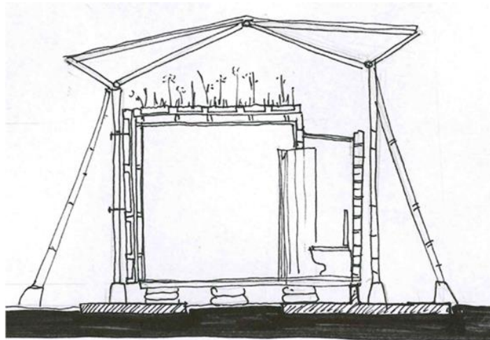
CORTE TRANSVERSAL
