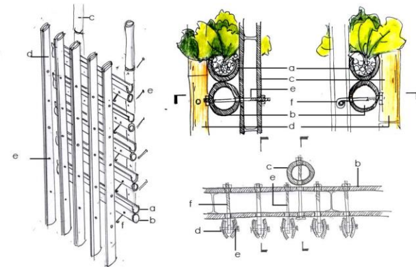
esquema funcionamiento
