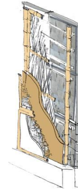
A- Fabricación y montaje de envolventes multiestrato
