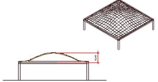
Detalles constructivos de la cúpula y el muro de adobe reforzado. Fuente: Barrionuevo 2011 .
