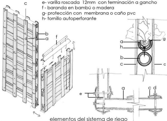
elementos del sistema de riego
