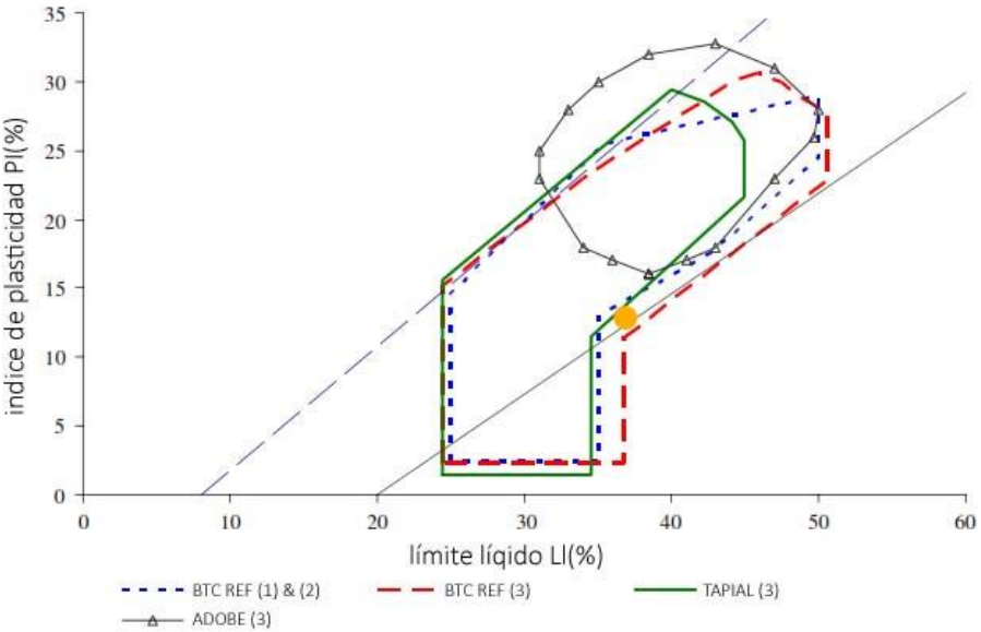
Gráfico 5: Diagrama que delimita el área de distribución de partículas según las distintas técnicas: Adobe, Bloques BTC y Tapiales. Referencias: AFNOR XP-P13 901 [1], CRATerre (ARSO) [2], Houben [3]
