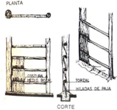
Detalles de la colocación de chorizos de paja y tierra. fuente: TIPOS PREDOMINANTES DE LA VIVIENDA RURAL EN ARGENTINA, FADU-UBA 1983
