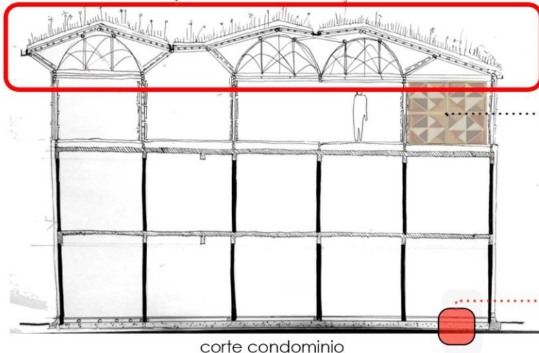
panel en bambú con revoque en tierra
