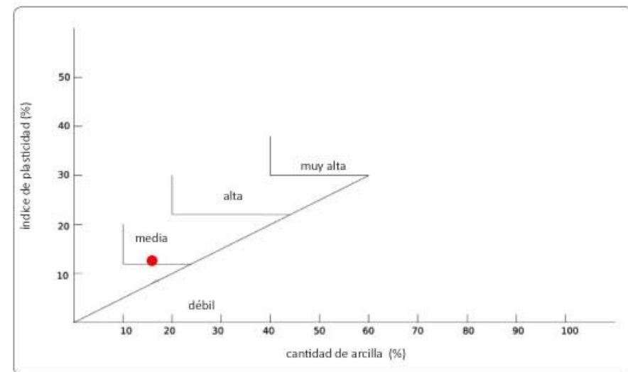
Gráfico 4: Expansión, grado de expansión de la tierra en relación a los límites de Atterberg. Fuente: Houben, Guillaud 1994
