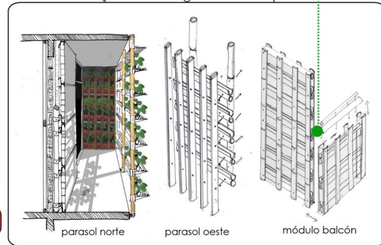
paneles de agricultura hidróponica
