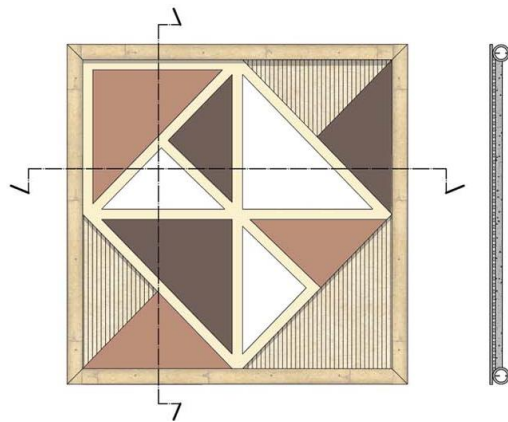
Proyecto para panel en bambú revocado con tierra, y pruebas de degrado.
