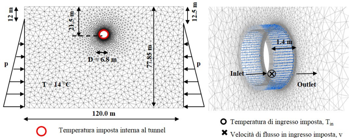
Fig 2. Geometria e dimensioni del modello 3D.
