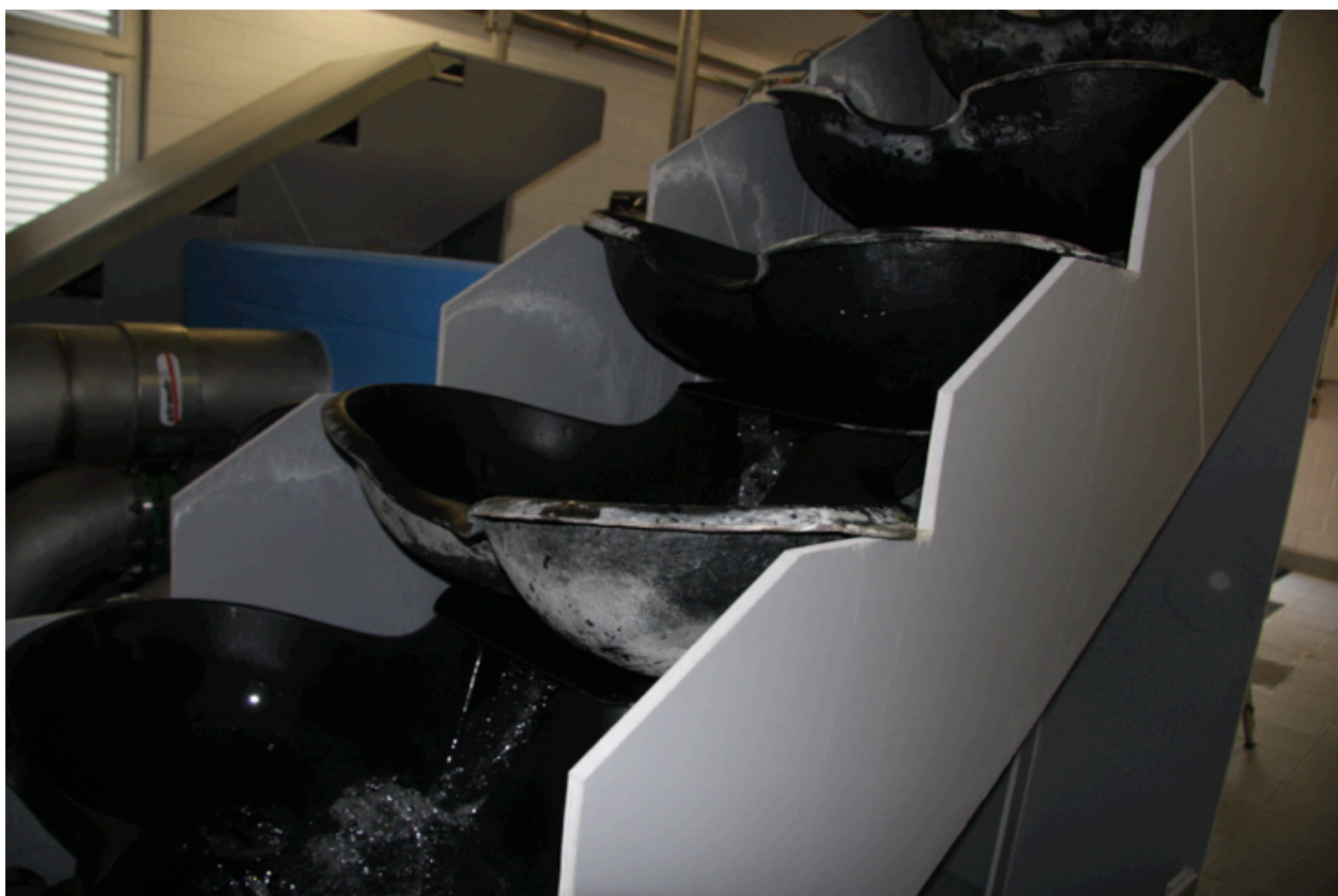
Sistema di Flow Form composto da 2 batterie di 5 vasche ciascuna in uscita dalla turbina
