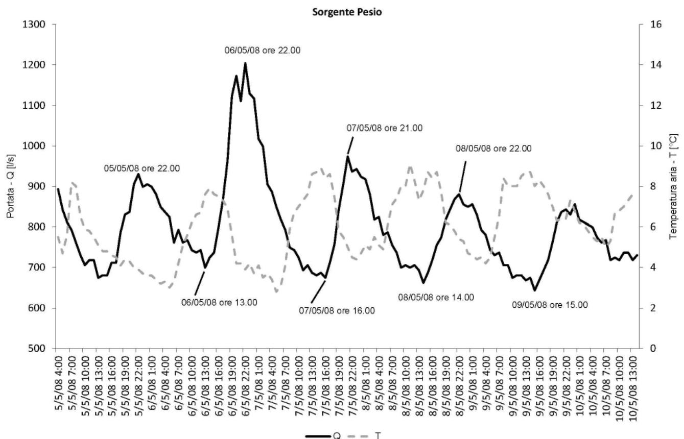
Fig. 2. Andamento giornaliero della portata di una sorgente alimentata dal processo di fusione nivale. In tratteggio la temperatura dell'aria (Sorgente del Pesio, Valle Pesio, CN).
