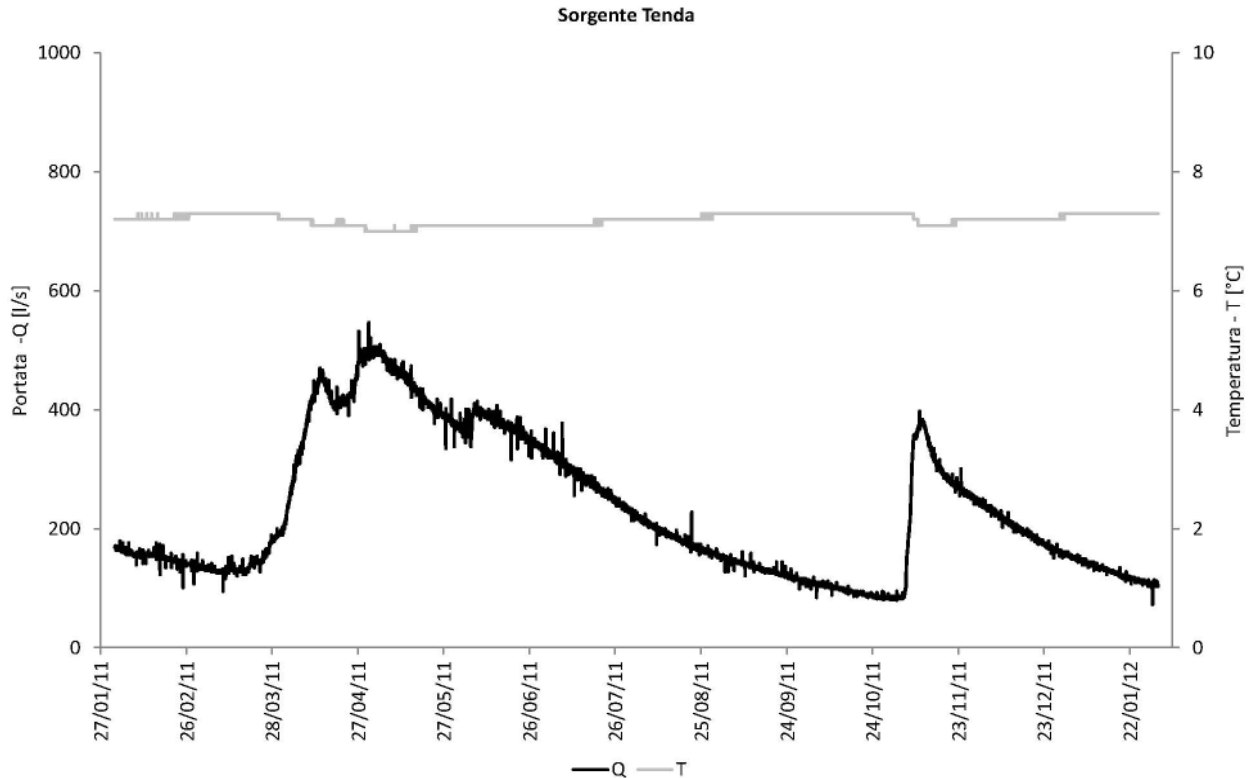
Fig. 11. Andamento annuale della portata e della temperatura delle acque di un sistema con alimentazione primaria prevalente. (Sorgente del Colle di Tenda, Valle Vermenagna, CN). Annual trend of flow rate and temperature of spring water fed by a prevalent primary input (Colle di Tenda spring, Vermenagna Valley, CN).
