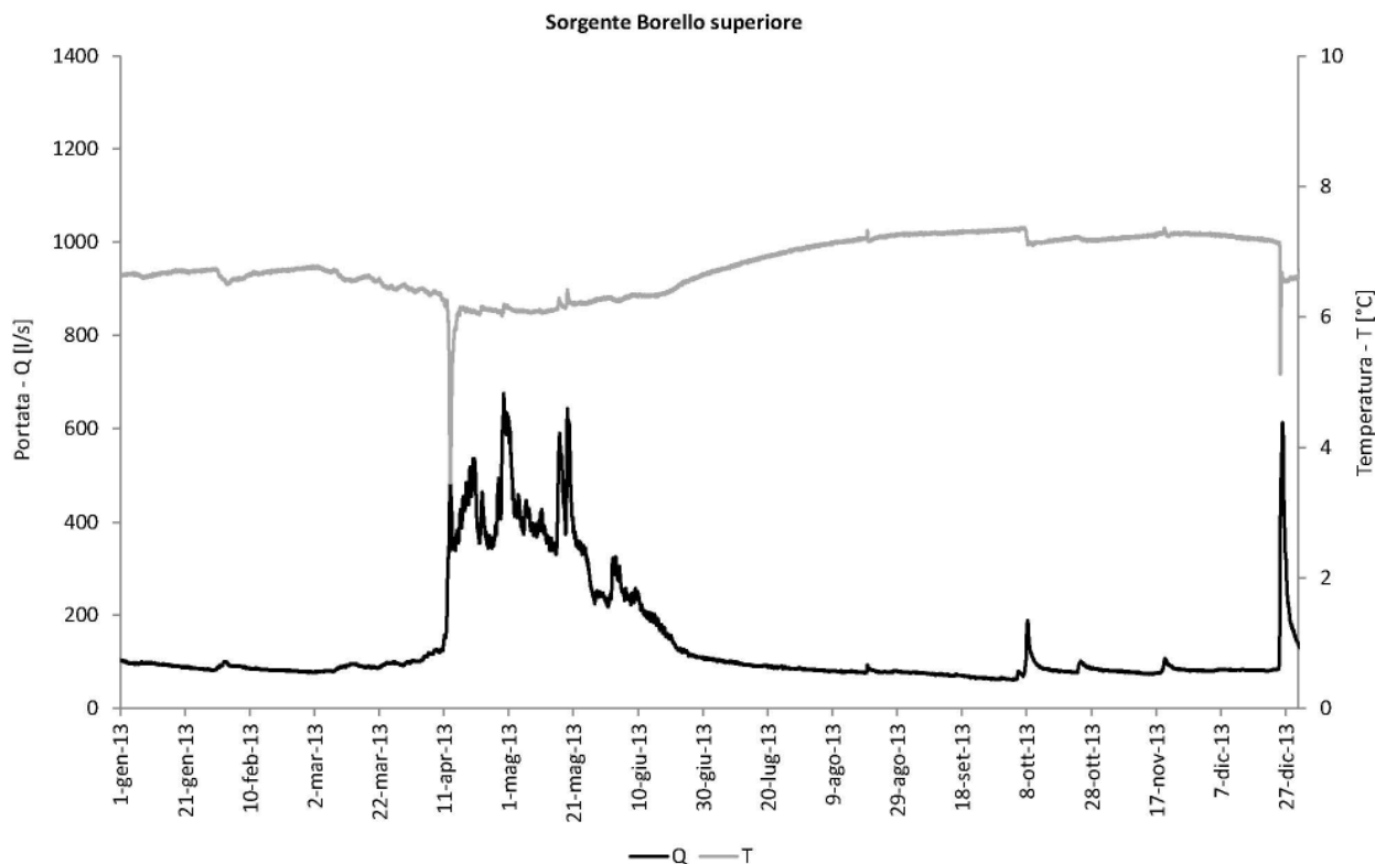
Fig. 12. Andamento annuale della portata e della temperatura delle acque di un sistema con alimentazione primaria e secondaria. (Sorgente di Borello Superiore, Valle Corsaglia, CN).
