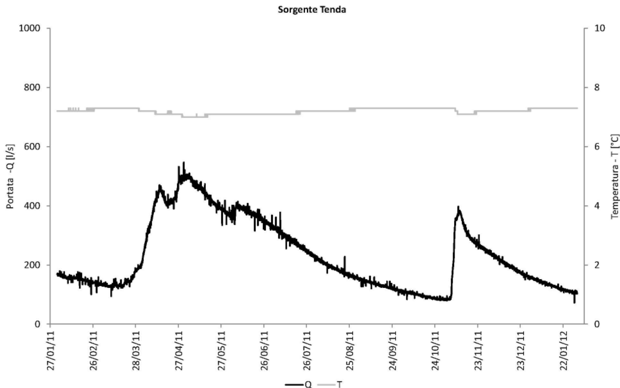
Fig. 11. Andamento annuale della portata e della temperatura delle acque di un sistema con alimentazione primaria prevalente. (Sorgente del Colle di Tenda, Valle Vermenagna, CN).
