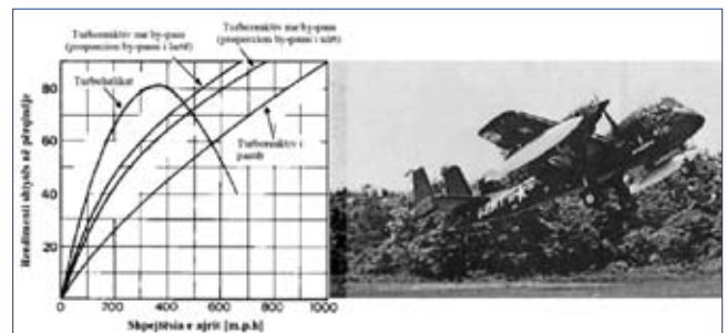
Figura 3. Rendimenti motorik në varësi të shpejtësisë së fluturimit ku shihet qartë rendimenti më i mirë i turbohelikave në shpejtësitë e ulta. Në të djathtë një avion Grumman OV1 Mohawk i pajisur me turbohelika, në një nisje STOL
