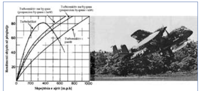
Figura 3. Rendimenti motorik në varësi të shpejtësisë së fluturimit ku shihet qartë rendimenti më i mirë i turbobelikave në shpejtësitë e ulta. Në të djathtë një avion Grumman OV1 Mohawk i pajisur me turbobelika, në një nisje STOL
