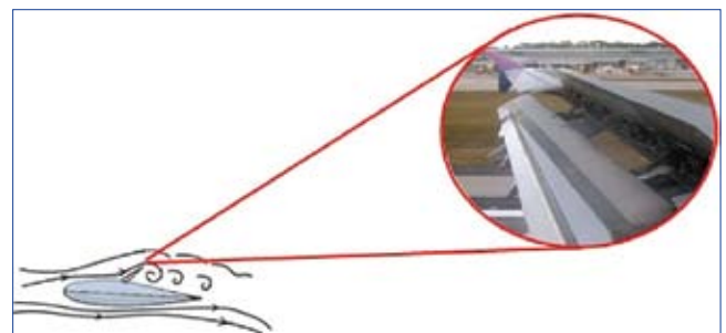
Figura 4. Efekti i spoilerave në krah, duke hequr forcën ngritëse dhe duke dhënë një efekt aerofrenues
