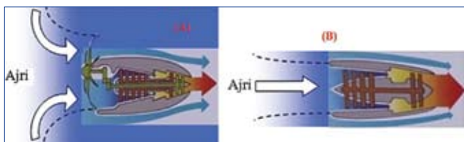
Figura 2. (A) Turbohelika ka një prurje ajri të madhe dhe pak të nxituar, (B) Turboreaktori ka një prurje ajri të reduktuar por shumë të nxituar
