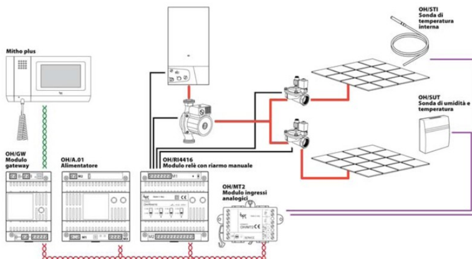
Fig. 1 - Esempio di impianto con 2 zone termiche con riscaldamento a pavimento, caldaia a condensazione, pompa e valvole idrauliche di zona ON/OFF con gestione del profilo settimanale della modalità automatica e del programma di controllo proporzionale (documentazione BPT).
