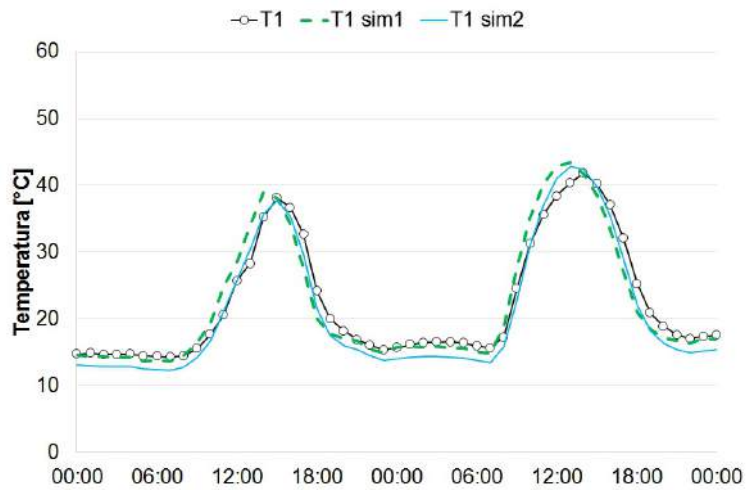
Figura 10.8: Temperatura superficiale esterna, t_1 , dati misurati e simulati, CScA. Con sim1 =risultati MATS, con sim2 =risultati F.Z.
