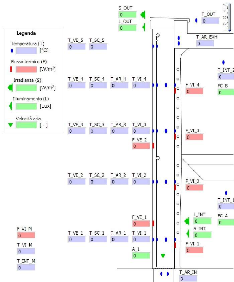
Figura 8.11: Schema dei sensori della facciata Somec, CSb.
