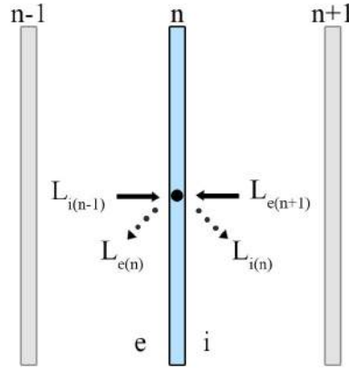
Figura 7.5: Bilancio short-wave sul nodo.
