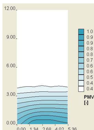
Figura 6.6: Esempio di mappa di valori di PMV in un ambiente testato con HyperComfort.
