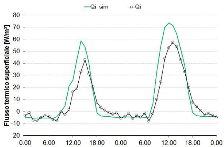
Figura 10.7: Flussi termici superficiali, dati misurati e simulati, CSa.
