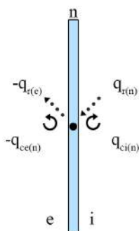
Figura 7.9: Bilancio sul nodo
