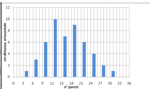
Figura 3. Grafico relativo all'irregolarità dei muri delle baite di Veglio. Sull'asse delle ordinate le distanze orizzontali [cm]; sull'asse delle ascisse la quantità di pareti presentanti la stessa irregolarità.
