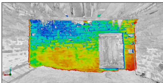
Figura 2. Visualizzazione dell'andamento della parete in relazione ad un piano verticale interpolante i punti del muro. Progressivamente dal rosso (punti di maggiore aggetto) al blu (punti di maggiore rientranza).
