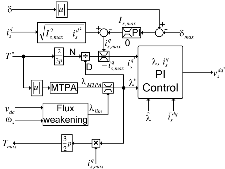
Fig. 3.15: UDFVC Scheme
