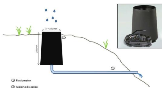
Figura 1 - Schema di pluviogramma interrato di nuova generazione.
