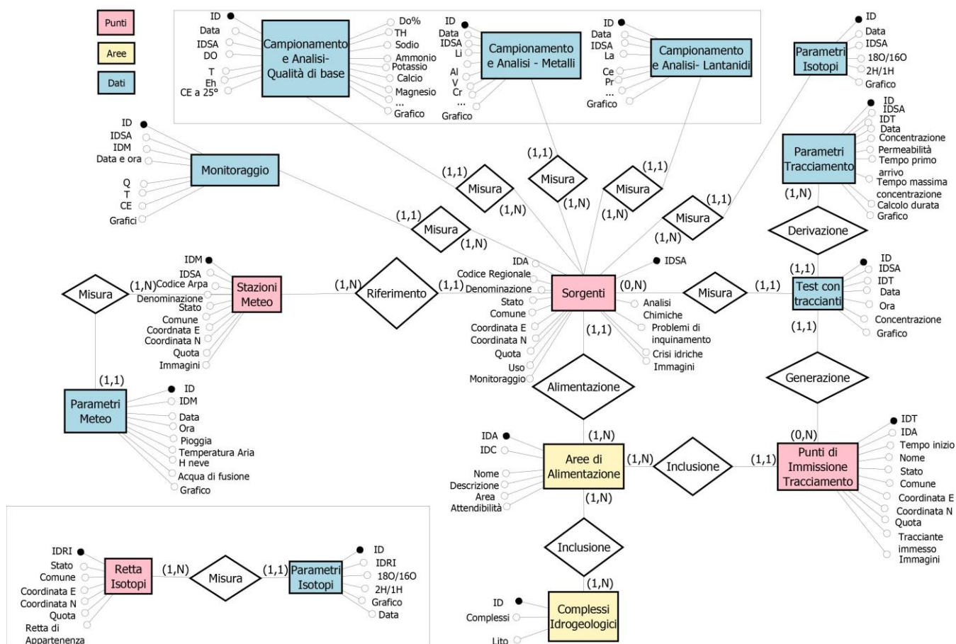
Figura 3 - Modello concettuale
