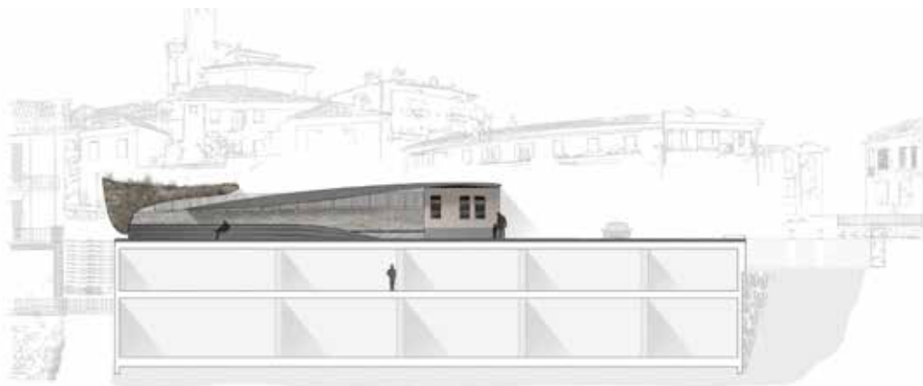
Sezione AA, scala 1:200 / Section AA scale 1:200
