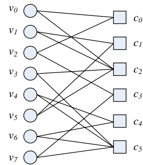
Fig. 5 Bipartite of LDPC codes.
