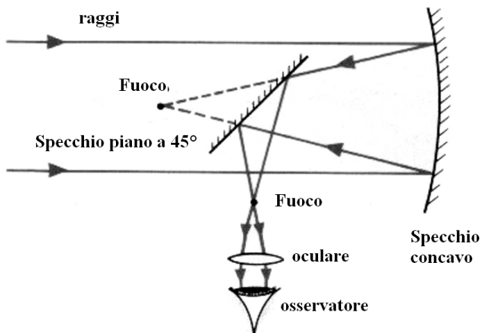
Schema del telescopio a riflessione di Newton, formato da uno specchio concavo, uno piano e un oculare.
