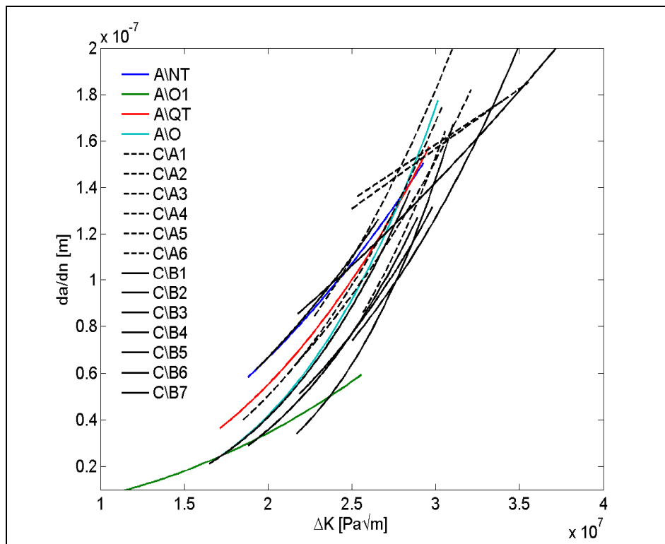
Fig. 60 – Curve di Paris valutate nel corso della precricatura (non valide secondo la norma E647).
