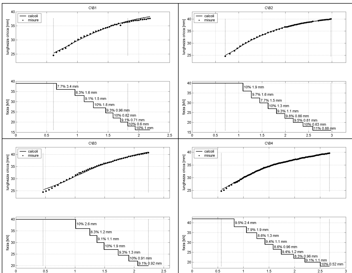
Fig. 73 – Cicli e carichi (ampiezze) impiegati ed avanzamenti di cricca misurati e calcolati nel corso della precricatura dei campioni per K_{Ic} originari provenienti dal blumo C. Prima parte: provette da C\B1 a C\B4.
