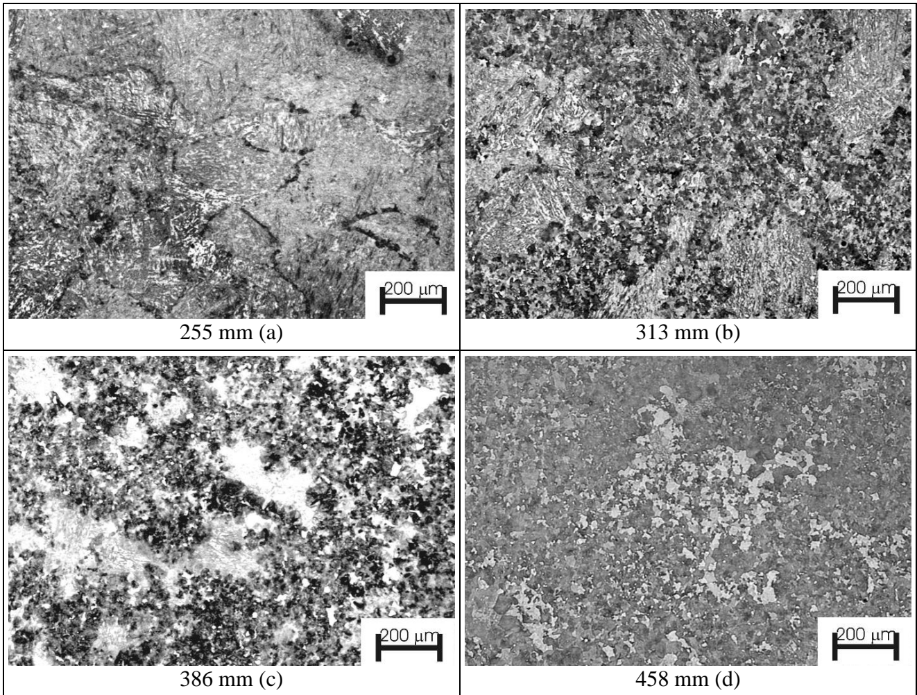
Fig. 29 - Blumo B, microstrutture a profondità crescenti. Piani ST. Microstruttura mista costituita da martensite e bainite rinvenute e da perlite fine localizzata presso i precedenti bordi di grano austenitici, a profondità 255 mm (a). Incremento graduale della frazione di perlite, a profondità 313, 386 e 442 mm (b,c,d). Campioni B\18 (a) , B\22 (b), B\27 (c) e B\32 (d). 126
