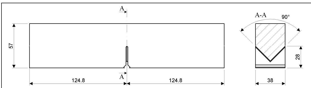
Fig. 69 – Disegno consuntivo della provetta A\O1. Le quattro facce maggiori sono state rettificare.
