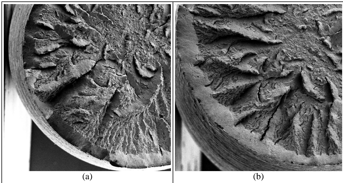
Fig. 45 – Campioni ritrattati termicamente (provenienti dal blumo C). Superfici di frattura dei campioni di trazione C\A1F (a) e C\A6C (b), osservati al microscopio elettronico a basso ingrandimento. Superfici di scorrimento di taglio (con tracce radiali) macroscopiche, simili a quelle osservate nella Fig. 44a. Le superfici di frattura sono totalmente costituite da microvuoti.
