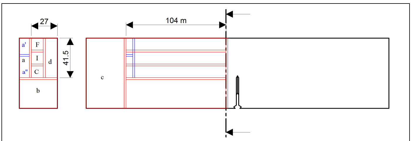
Fig. 40 – Prelievo di quadri di sezione approssimativa 12,5 x 12,5 mm, per la lavorazione di campioni di trazione, in diverse posizioni nei frammenti delle provette per K_{Ic} ritratte C\(\text{A}\text{n}\). I campioni sono stati denominati con i suffissi C (Cuore), I (Intermedio, poi non impiegati) ed F (Faccia). Nel caso C\(\text{A}4\), il frammento c si trovava presso il centro, anziché presso l'estremo, del campione per K_{Ic} . Le linee rosse e indicano i tagli eseguiti per ricavare detti quadri, le linee blu ulteriori tagli eseguiti per ricavare campioni metallografici e di durezza.
