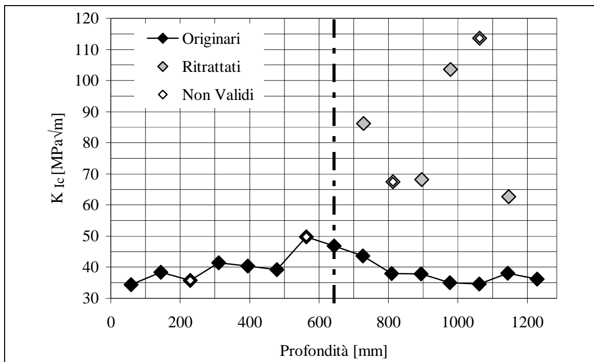
Fig. 18 – Misure di tenacità a frattura su provette provenienti dal blumo C, tali quali ricevute oppure ritratte, in funzione della profondità unilaterale originaria. Le misure su campioni originari a profondità (unilaterale) superiore a 600 mm sono state eseguite da ricercatori del Politecnico di Milano 125 .
