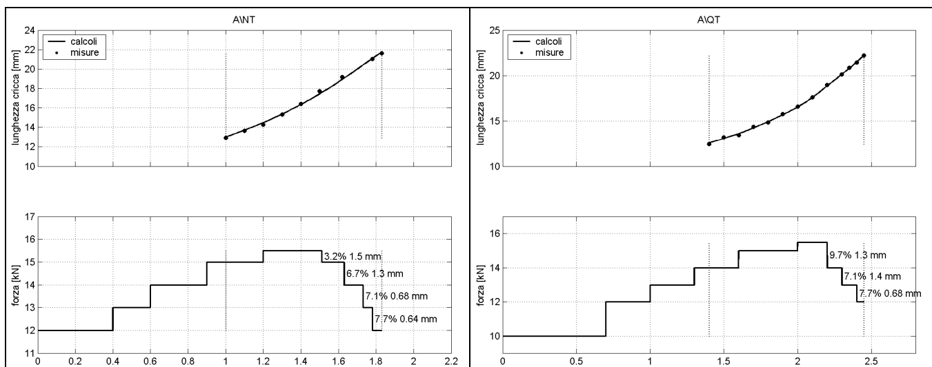
Fig. 75 – Cicli e carichi (ampiezze) impiegati ed avanzamenti di cricca misurati e calcolati nel corso della precriccatura dei campioni per K_{Ic} ritrattati provenienti dal blumo A.
