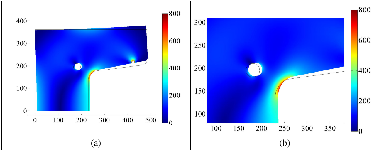
Fig. 4 - Analisi strutturale elastica in deformazione piana ad elementi finiti di parte della sezione di un punzone, disegnata in Fig. 3. Dimensioni in mm, tensioni equivalenti di Von Mises in MPa. Vista completa del modello (a) e dettaglio del raccordo (b). Codice di calcolo Femlab.*
