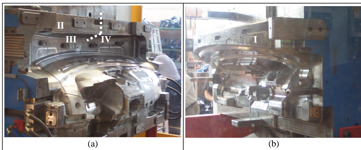
Fig. 2 – Punzone (a) e matrice (b) di uno stampo per la formatura di plance automobilistiche.
