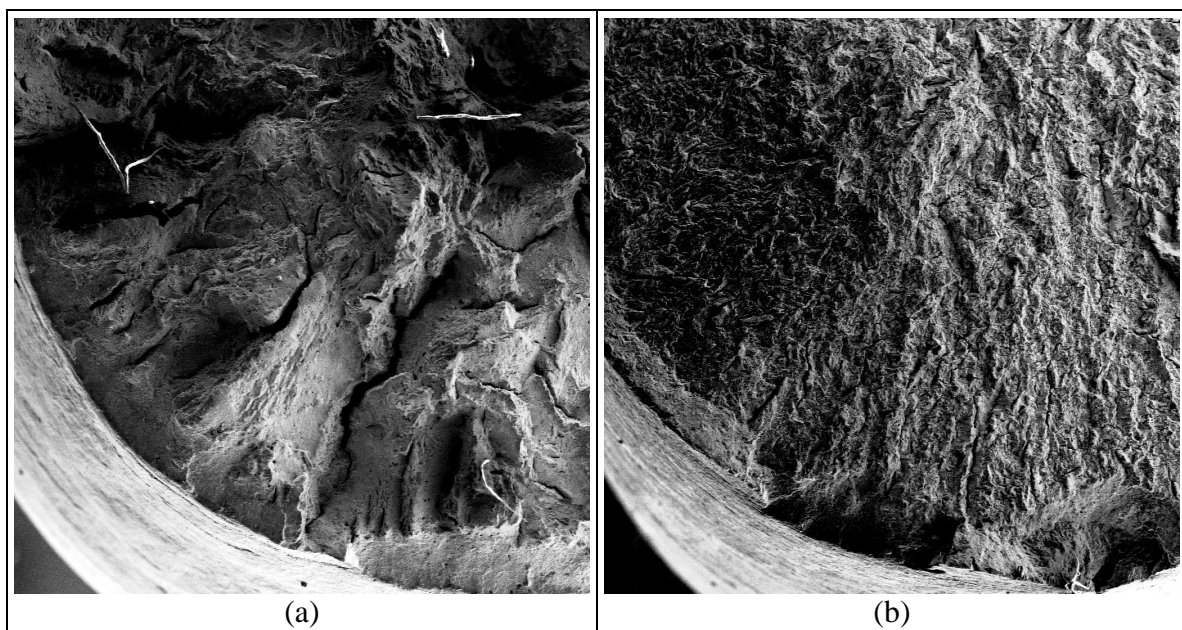
Fig. 44 – Blumo B. Superfici di frattura di campioni di trazione ricavati da profondità 65 mm (a) e 442 mm (cuore, b), osservati al microscopio elettronico a basso ingrandimento (uguale nei due casi). Diametro strizionato 5 mm (a) e 6 mm (b). Superfici di scorrimento di taglio macroscopiche (su una scala di 1 mm, con tracce radiali), evidenti nel campione proveniente dalla profondità minore (a). Le superfici di frattura sono totalmente costituite da microvuoti, in entrambi i casi.
