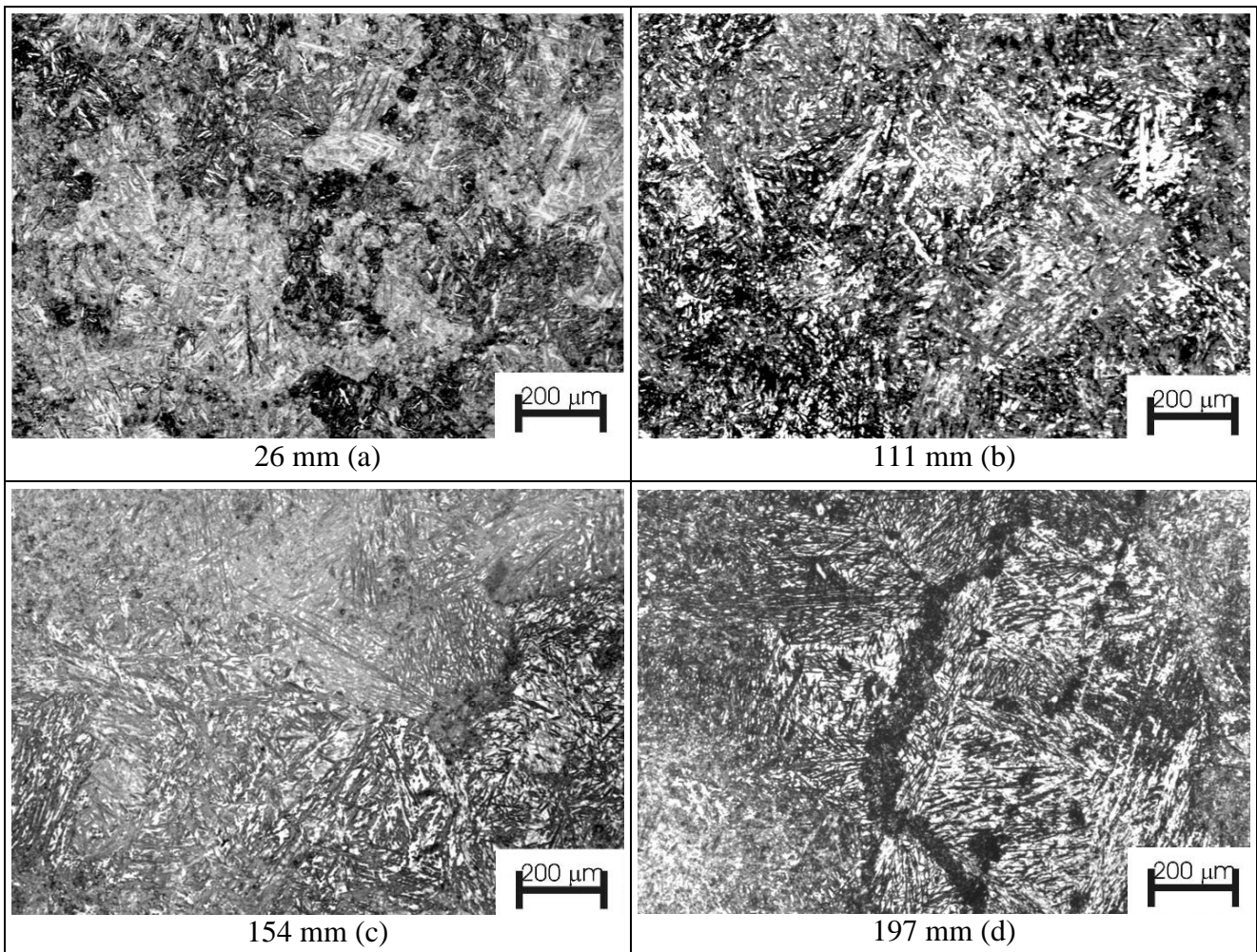
Fig. 28 - Blumo B, microstrutture a profondità crescenti. Piani ST. Microstruttura mista costituita da martensite e bainite rinvenute, a profondità 26 e 111 mm (a, b). Perlite presso e precedenti bordi di grano austenitici e conseguente segregazione composizionale, a profondità 154 e 197 mm (c,d). Campioni B\1 (a) , B\7 (b), B\11 (c) e B\14 (d). 126
