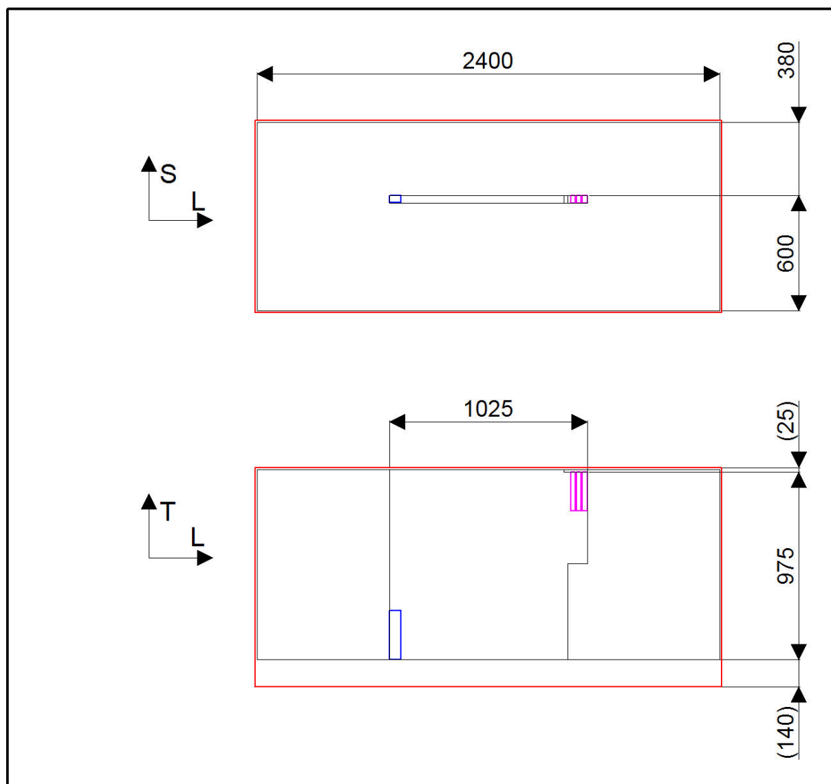
Fig. 14 – Campionamento del blumo A. Superfici temprate e rinvenute (rosso), superfici del blumo alla consegna e lastra utilizzata per il prelievo dei campioni (nero); campione A\O1 (blu) e campioni A\O, A\QT ed A\NT (viola). Quote in mm. Le quote 140 e 25 sono state stimate in base alla consuetudine industriale ed alle microstrutture osservate. Le dimensioni del campione A\O1 nelle direzioni L, T ed S sono 58, 255 e 38 mm rispettivamente; le corrispondenti dimensioni degli altri tre campioni sono 25, 200 e 41 mm. La scala è uguale a quella delle successive Fig. 15 e Fig. 16.
