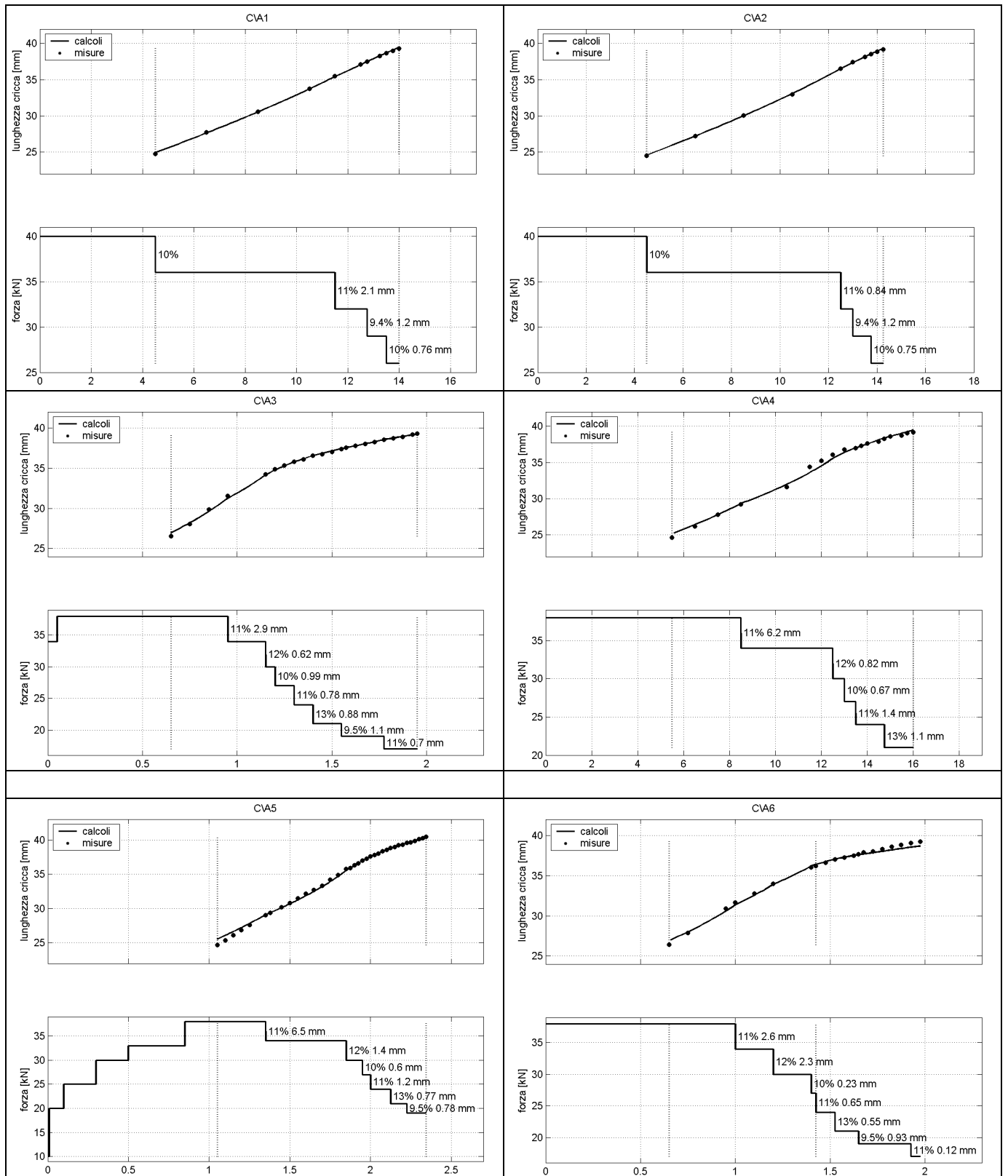
Fig. 76 – Cicli e carichi (ampiezze) impiegati ed avanzamenti di cricca misurati e calcolati nel corso della precricatura dei campioni per K_{Ic} ritrattati provenienti dal blumo C.
