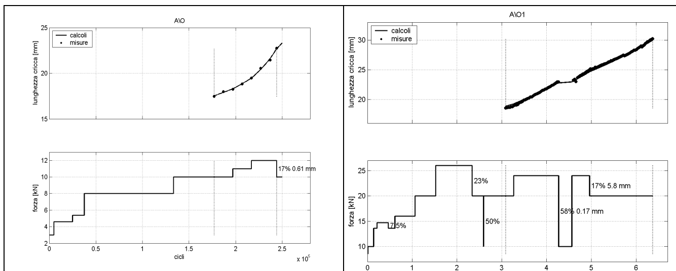
Fig. 72 – Cicli e carichi (ampiezze) impiegati ed avanzamenti di cricca misurati e calcolati nel corso della precricatura dei campioni per K_{Ic} originari provenienti dal blumo A.
