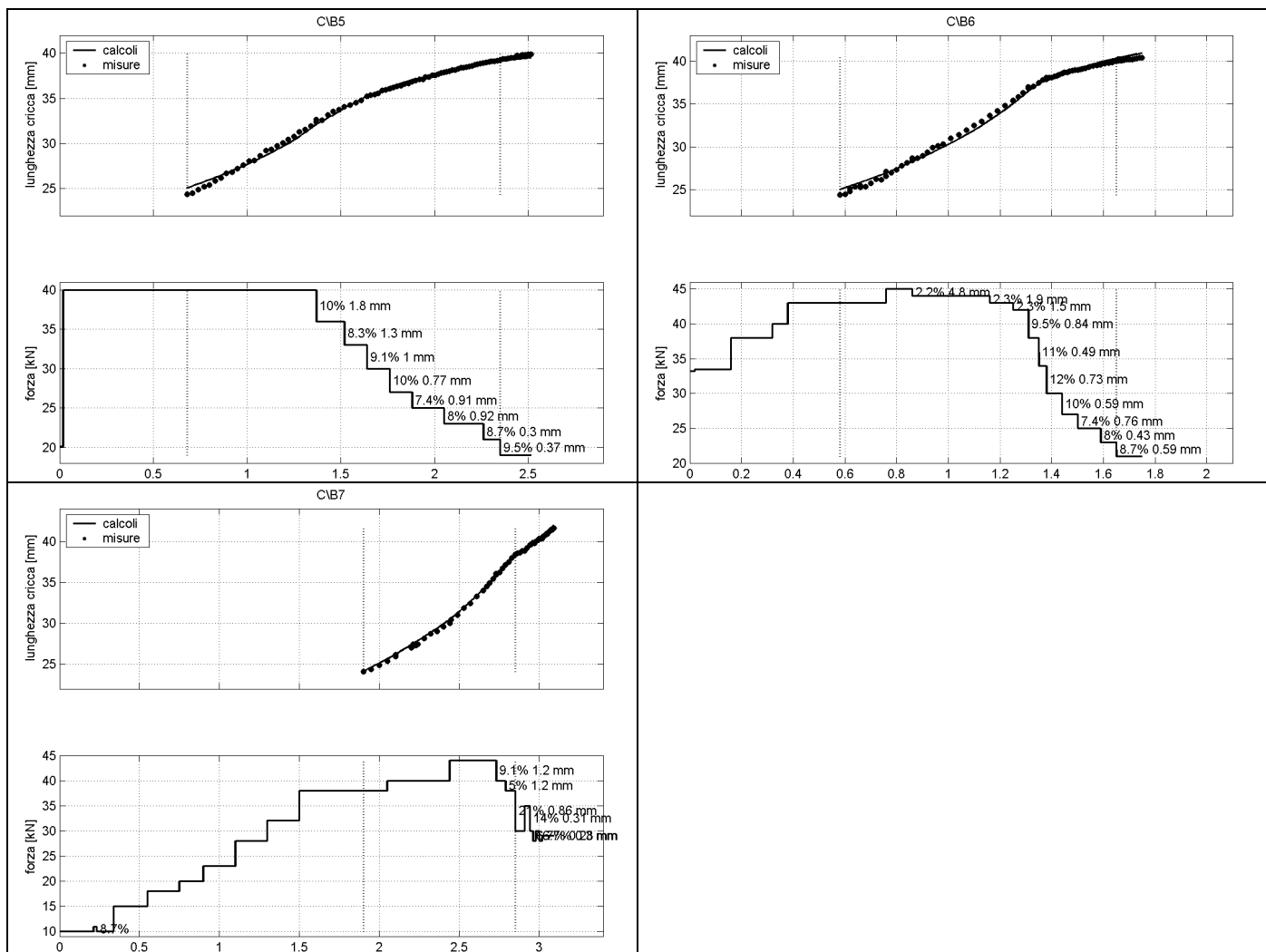
Fig. 74 – Cicli e carichi (ampiezze) impiegati ed avanzamenti di cricca misurati e calcolati nel corso della precriccatura dei campioni per K_{Ic} originari provenienti dal blumo C. Seconda parte: provette da CIB5 a CIB7.
