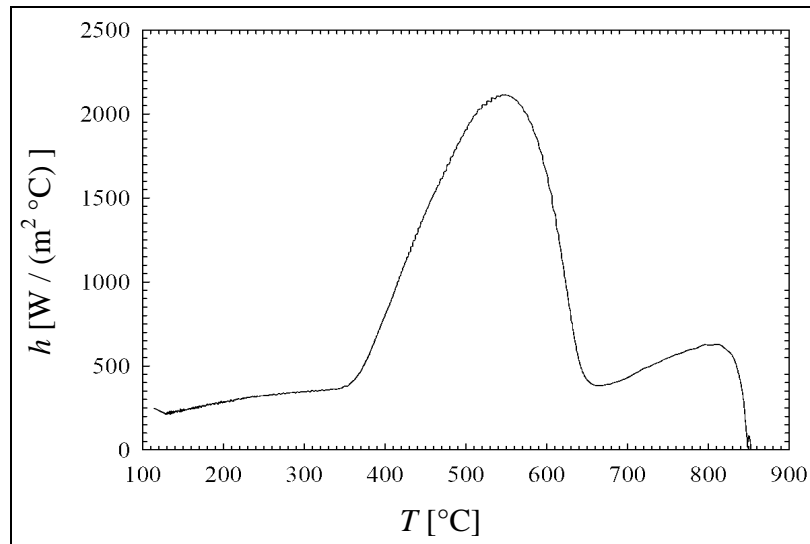
Fig. 80 – Coefficiente di scambio termico lineare h di un olio di tempra. 77
