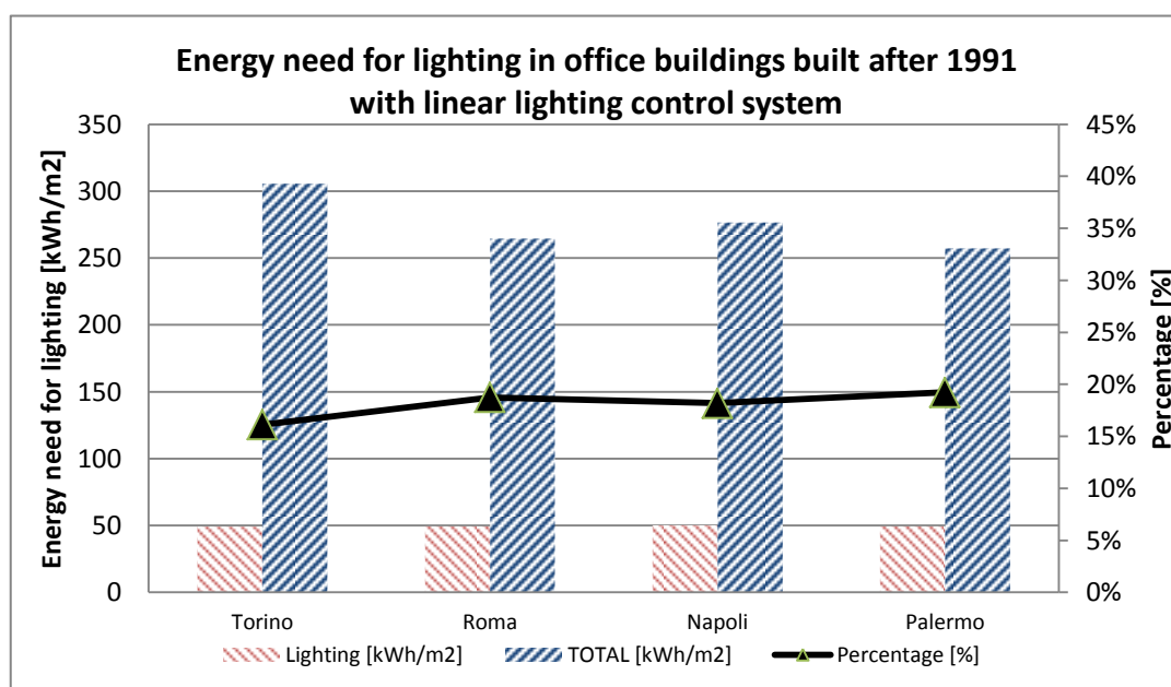
Figura 22 - Fabbisogno energetico per illuminazione e totale per edifici con controllo lineare costruiti dopo 1991
