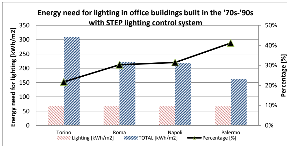
Figura 17 - Fabbisogno energetico per illuminazione e totale per edifici con controllo non lineare costruiti nel periodo 1970-1990
