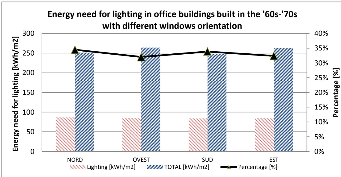
Figura 25 - Fabbisogno energetico per illuminazione e totale per edifici costruiti nel periodo '60 -'70 con finestre diversamente orientate
