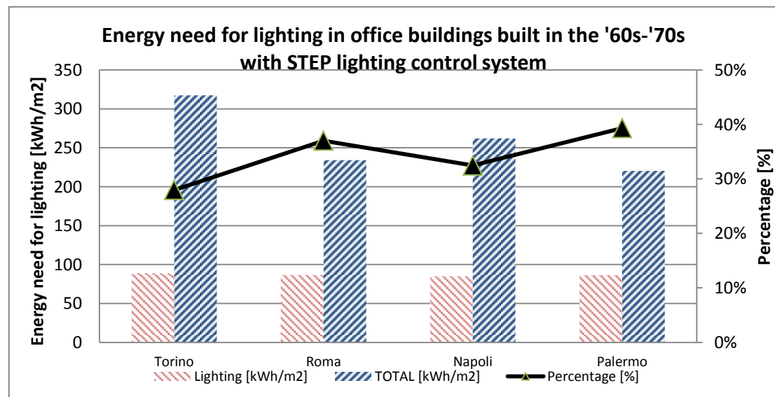
Figura 16 - Fabbisogno energetico per illuminazione e totale per edifici con controllo non lineare costruiti negli anni '60-'70
