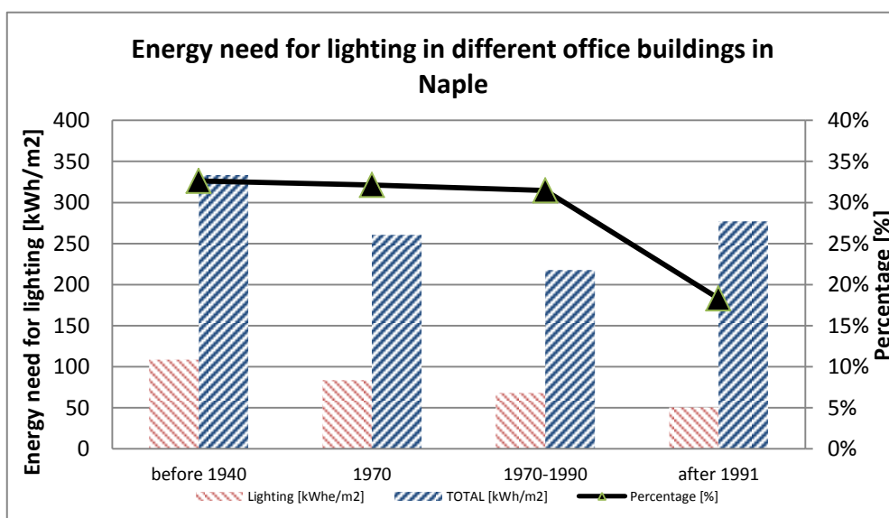
Figura 7 - Fabbisogno energetico per illuminazione e totale per le diverse tipologie di edifici per uffici a Napoli
