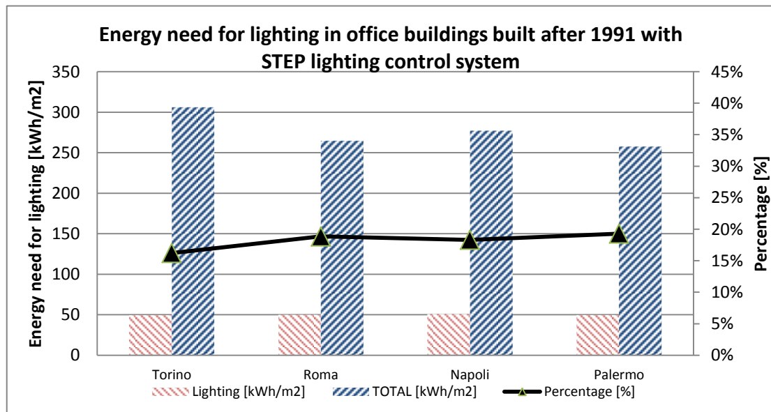
Figura 18 - Fabbisogno energetico per illuminazione e totale per edifici con controllo non lineare costruiti dopo 1991
