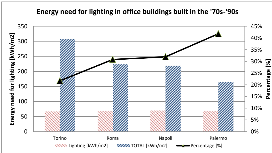
Figura 11 - Fabbisogno energetico per illuminazione e totale per edifici costruiti nel periodo 1970-1990
