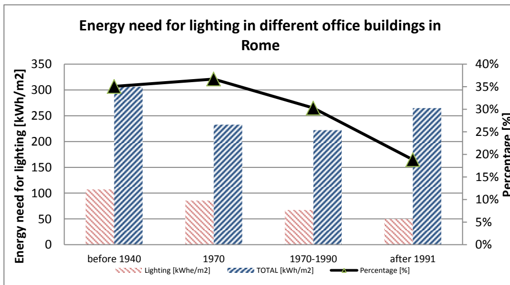
Figura 6 - Fabbisogno energetico per illuminazione e totale per le diverse tipologie di edifici per uffici a Roma
