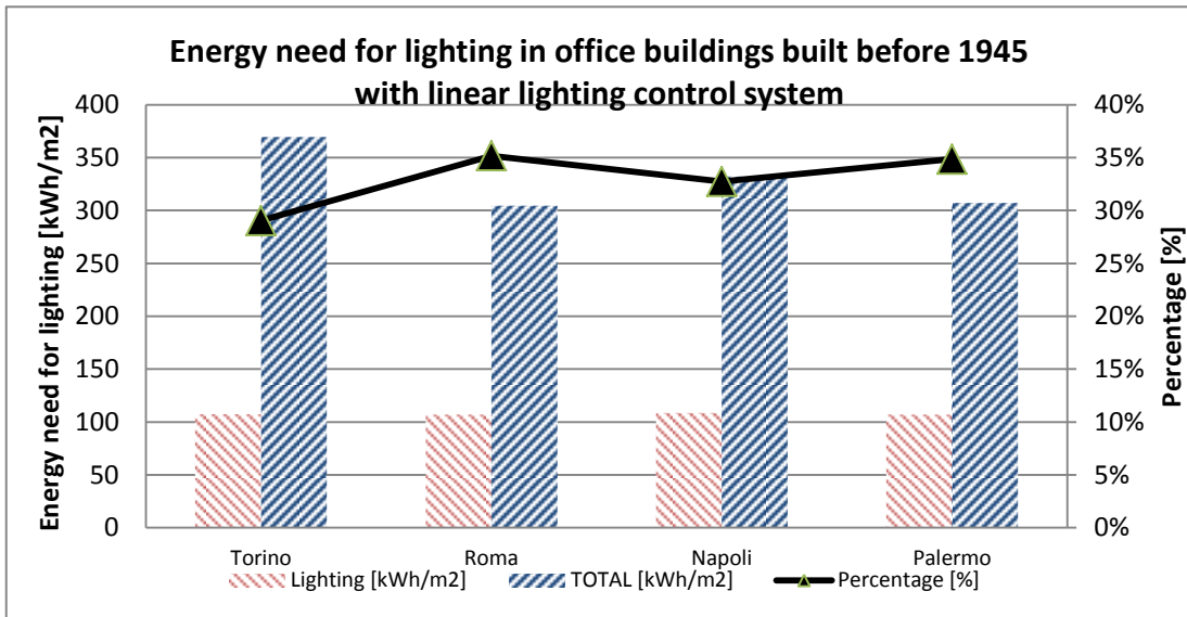
Figura 19 - Fabbisogno energetico per illuminazione e totale per edifici con controllo lineare costruiti prima del 1945
