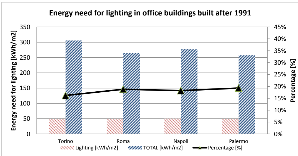
Figura 12 - Fabbisogno energetico per illuminazione e totale per edifici costruiti dopo il 1991
