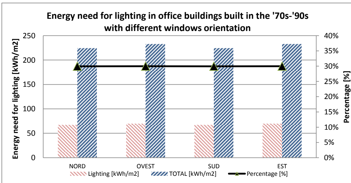
Figura 26 - Fabbisogno energetico per illuminazione e totale per edifici costruiti nel periodo '70 -'90 con finestre diversamente orientate
