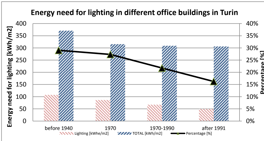
Figura 5 - Fabbisogno energetico per illuminazione e totale per le diverse tipologie di edifici per uffici a Torino
