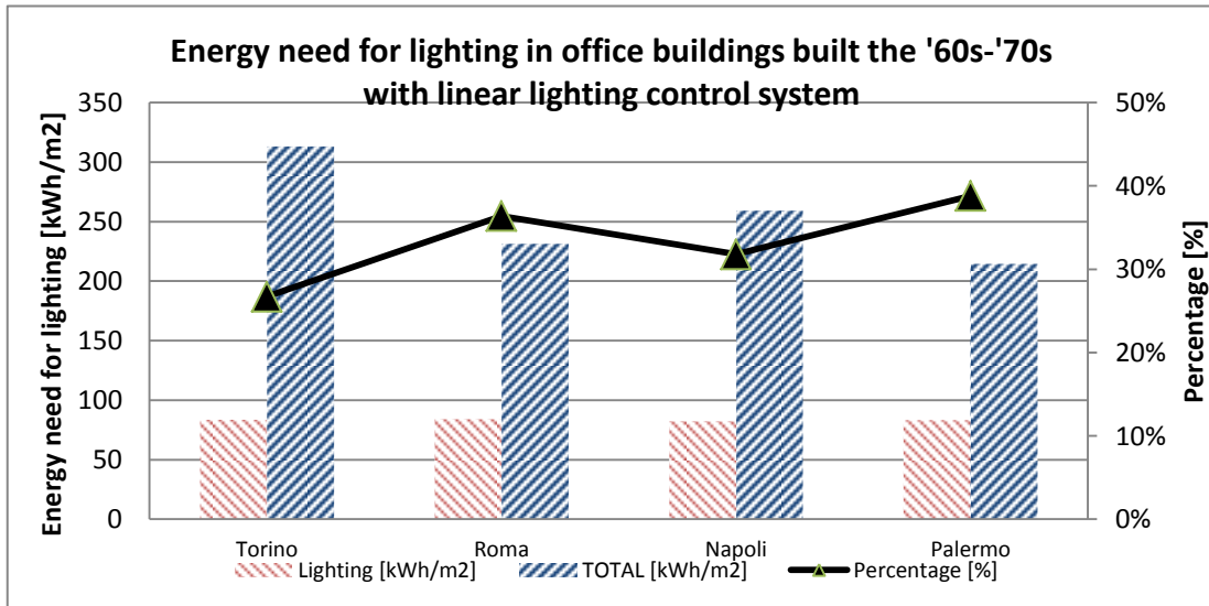
Figura 20 - Fabbisogno energetico per illuminazione e totale per edifici con controllo lineare costruiti negli anni '60-'70
