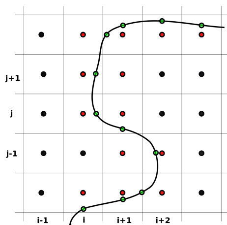
Figure 3.2: Classification des points du maillage : les points réguliers sont en noir, les points d'interface sont en rouge et les intersections sont en vert. Les lignes continues entourent les cellules.
