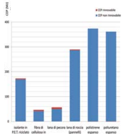
01 | L'istogramma confronta il Contenuto di Energia Primaria concernente l'isolamento termico di un involucro edilizio opaco. I dati si riferiscono all'energia necessaria per ottenere una trasmittanza termica di 0,24 W/m 2 K in una parete esterna verticale
