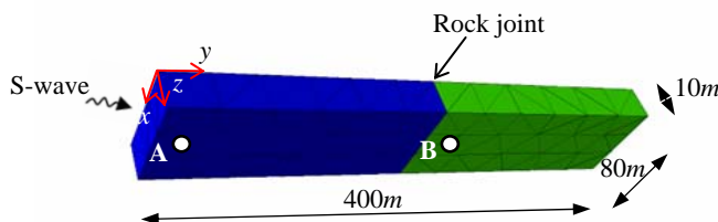
Figura 1. Modello 3DEC della colonna contenente un giunto in mezzeria
