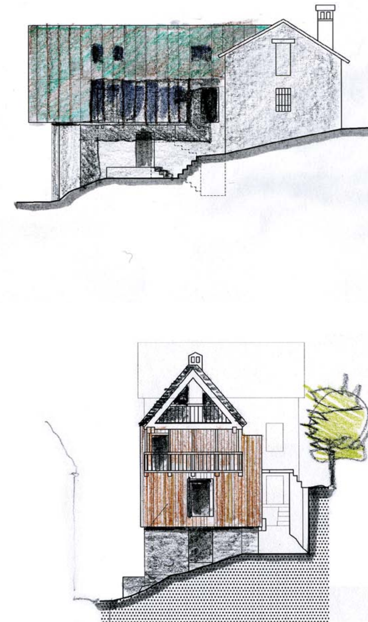
[Fig. 22 - Ranco - isolamento termico a cappotto esterno rivestito in legno locale non trattato - scala: 1:200]
