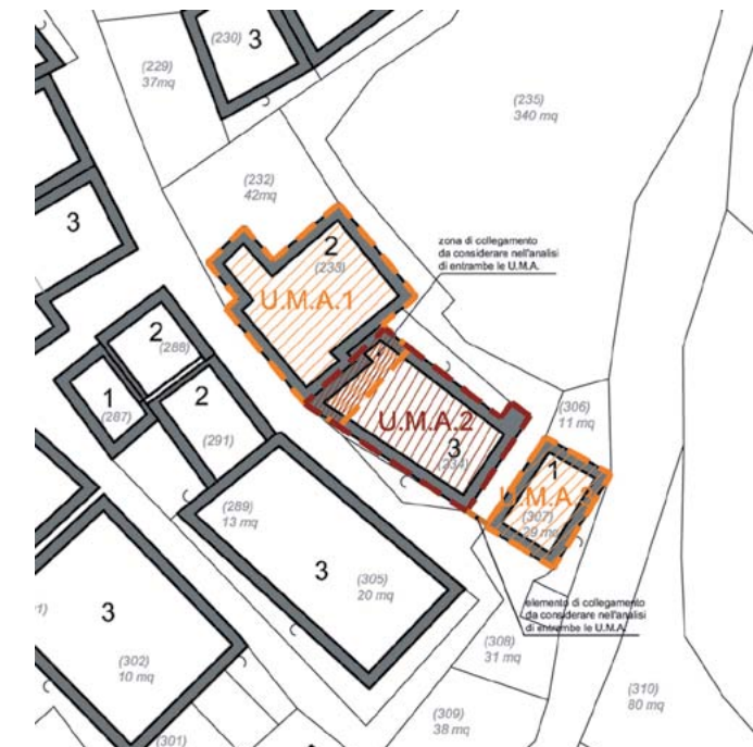
[Fig. 19 - individuazione dell'unità minima di analisi - Scala 1:500]
