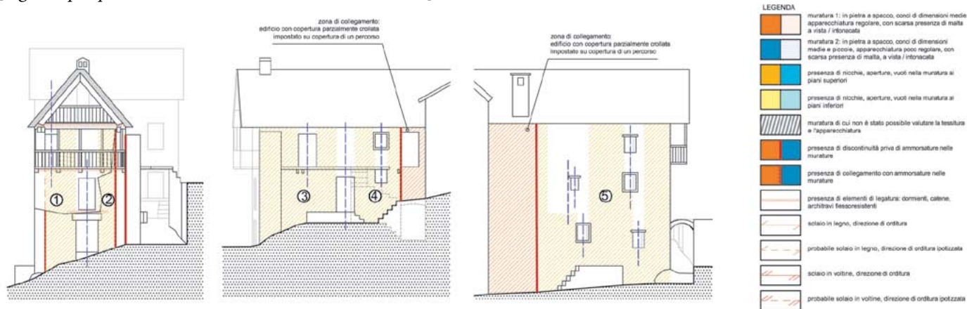
[Fig. 21 - prospetti sud-est, nord-est, sud-ovest - scala 1:200]
