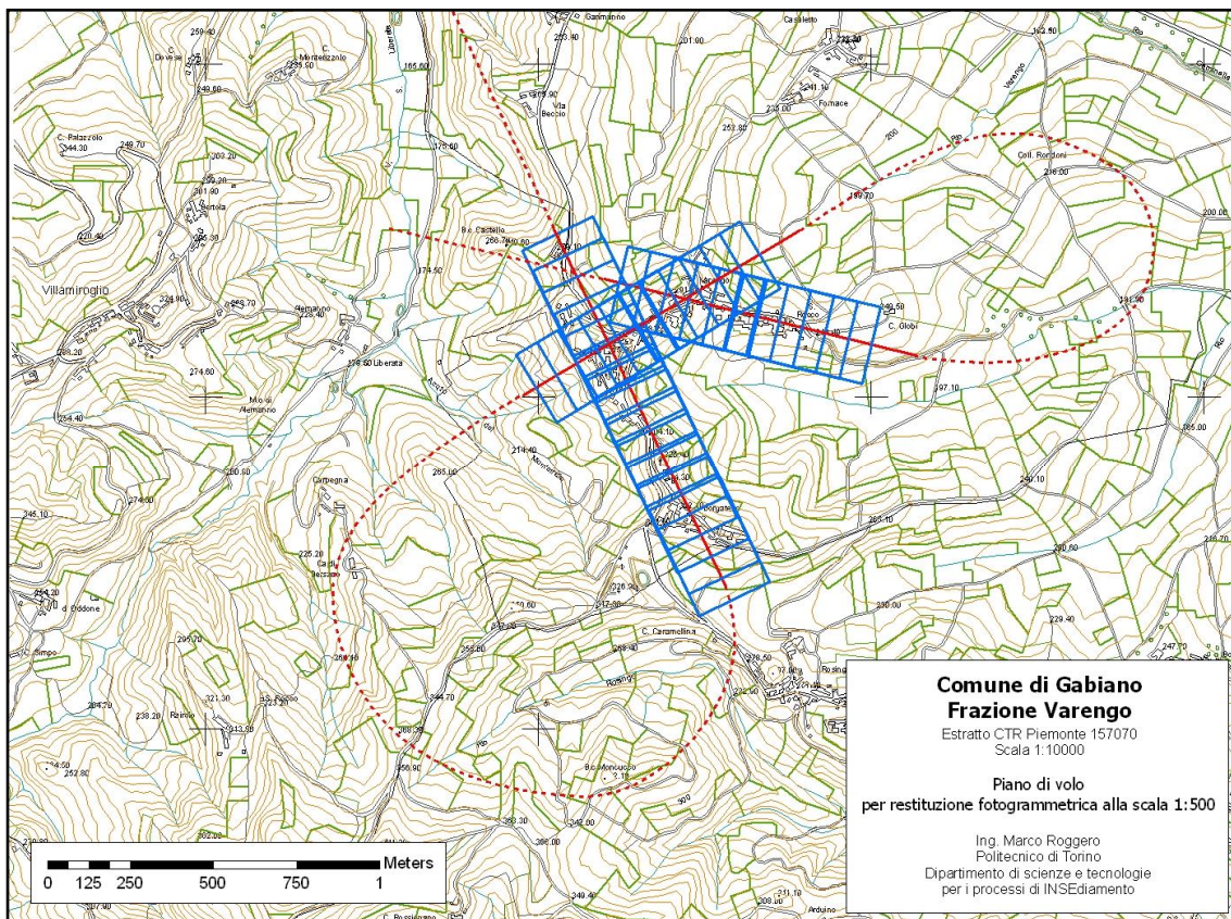
Fig. 8 – Piano di volo per la copertura fotogrammetrica alla scala 1:500 della frazione Varenco.
