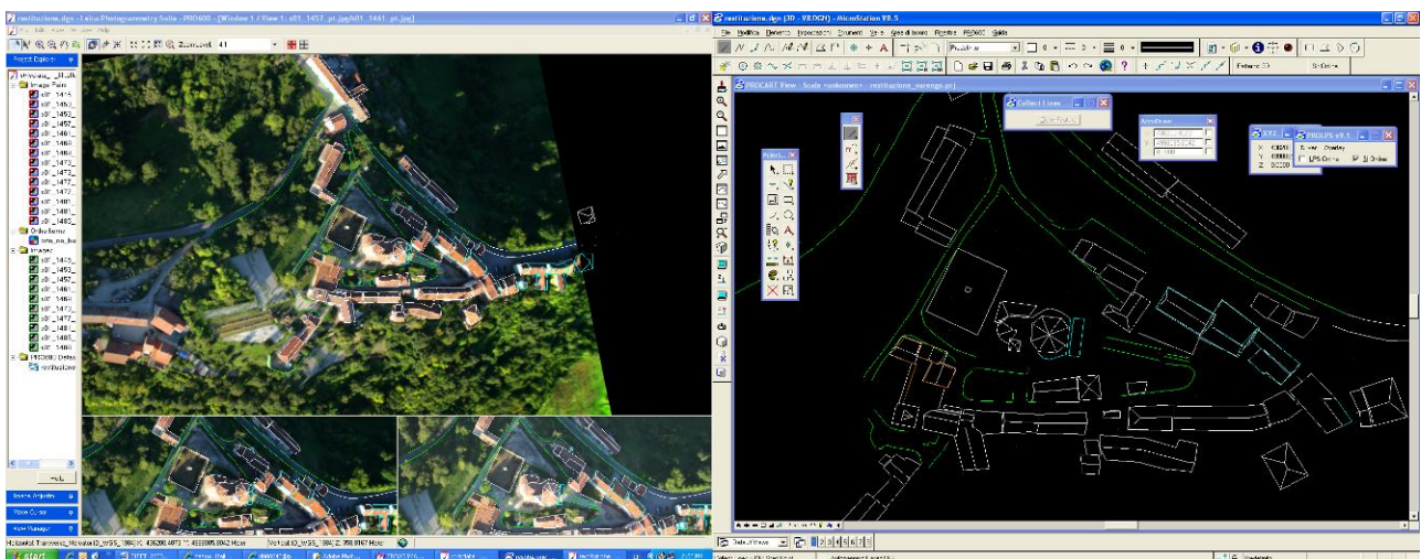
Fig. 12 - Fasi di restituzione nel modulo PRO-600 del software Leica Photogrammetric Suite
