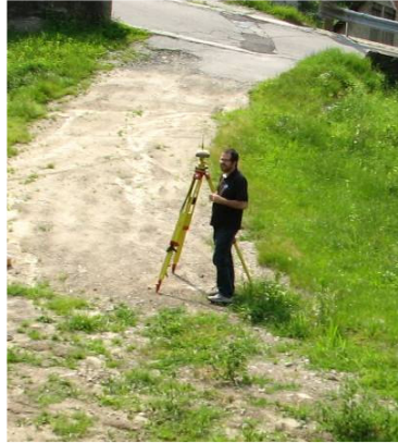
Figura 2 – stazione master
