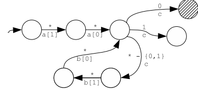
(a) Template automaton
