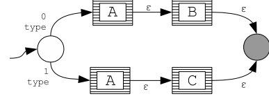
(d) FSA for the switch construct
