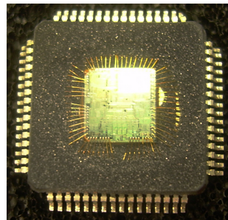
Fig. 6 DUT photo.
