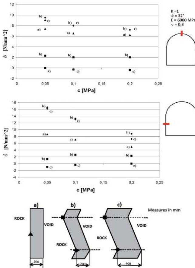
Fig. 8. Stresses computed at the estradosso of the tunnel for K=1 vs cohesion of the rock mass – Case B. Tensioni calcolate all'estradosso del tunnel per K=1 al variare della coesione della roccia – Caso B.
