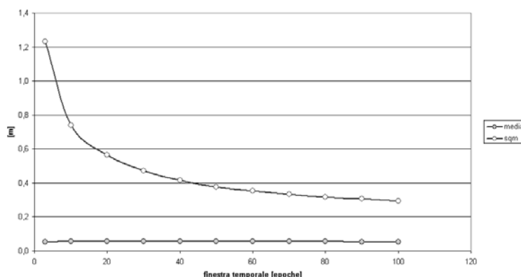
Fig 7 - medie e sqm in \phi nel posizionamento differenziale a Torino al variare della finestra.
