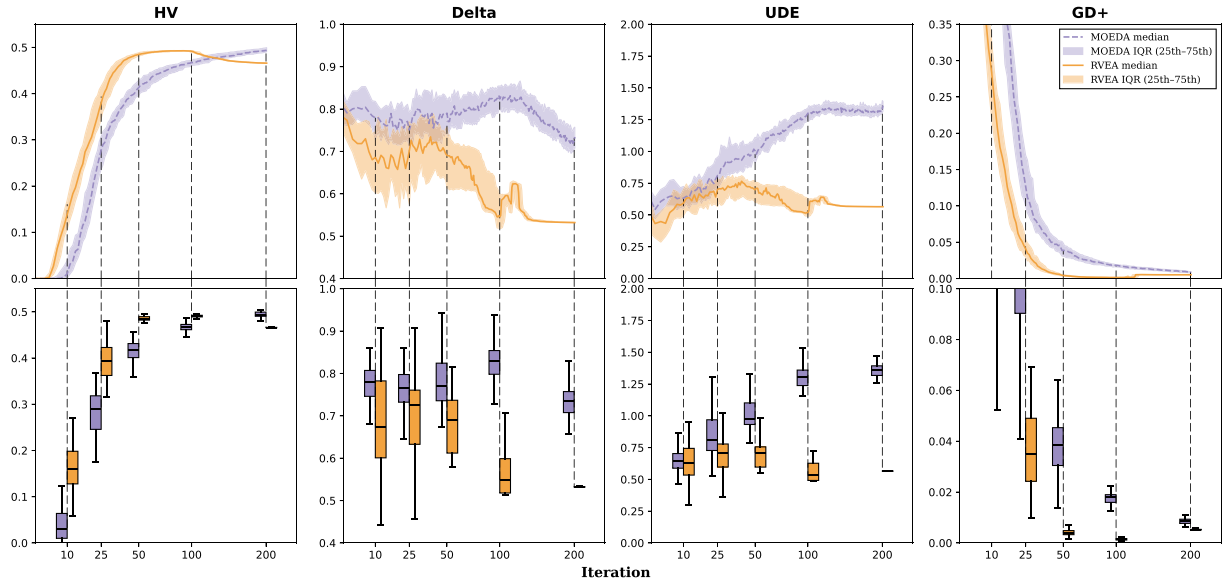
Fig. 26. ZDT3: MOEDA-GMM champion vs RVEA.
