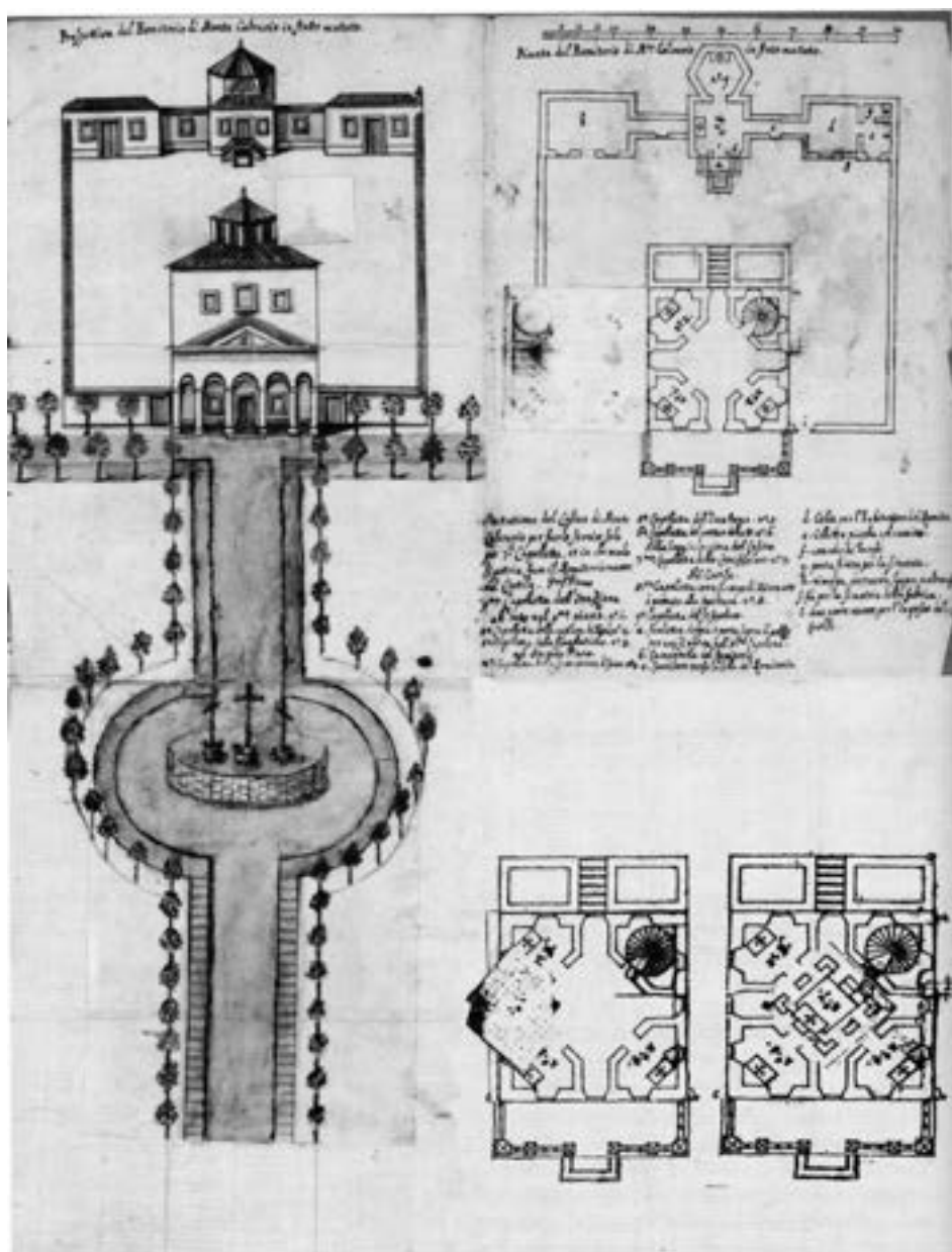
Fig. 11. Santo Deserto di Monteverginio, Progetto di ampliamento del romitorio del Monte Calvario e della cordonata di accesso: vista a volo d'uccello, piante del piano terreno, del primo e secondo piano, penna e acquerello, fine sec. XVII (Roma, Archivio di Stato, Carmelitani Scalzi, S. Maria della Vittoria, fasc. 524, n. 10).
