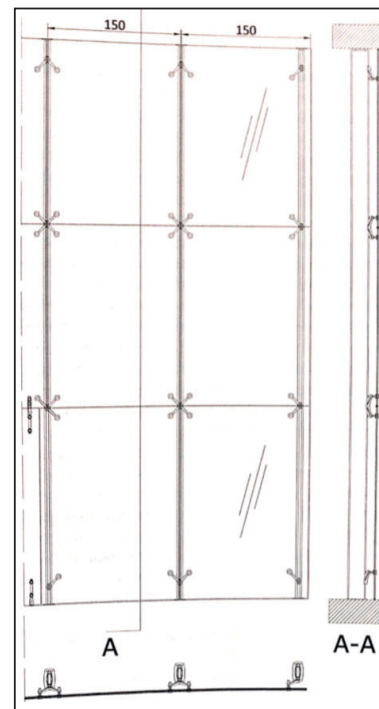
Sezioni e prospetto di una vetrata con dispositivi di fissaggio a crociera da Campioli A., Lavagna M., Tecniche e architettura , Città Studi
