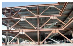
Telaio in acciaio da https://unikore.it/phocadownload/userupload/tiziana.basirico-unikore.it/Arch_Tec_Lez_09_struf%20elevazione.pdf
