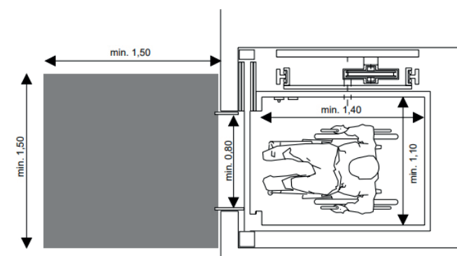
Esempi di spazi progettati secondo i principi di accessibilità da L. FANTINI e G. VENTURELLI, Progettare la normalità schede tecniche per una progettazione senza barriere , Maggioli Editore - Rimini
