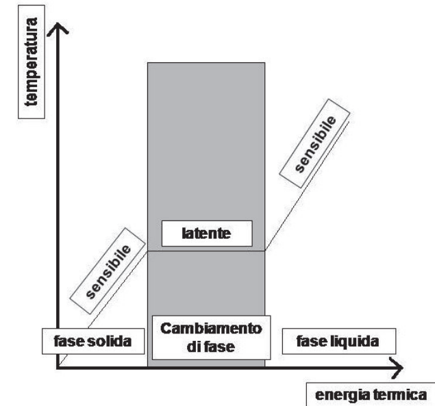
Schemi sui PCM da https://www.teknoring.com/guide/guide-edilizia-e-urbanistica/materiali-a-cambiamento-di-fase-in-edilizia-principi-e-applicazioni/
