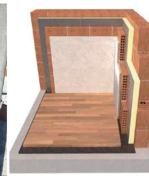
Isolamento termico in intercapedine da https://www.knaufinsulation.it/applicazioni/pareti-perimetrali
