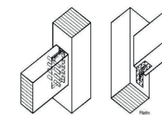
Incollaggi e chiodature da https://unikore.it/phocadownload/userupload/tiziana.basirico-unikore.it/Arch_Tec_Lez_09_struf%20elevazione.pdf
