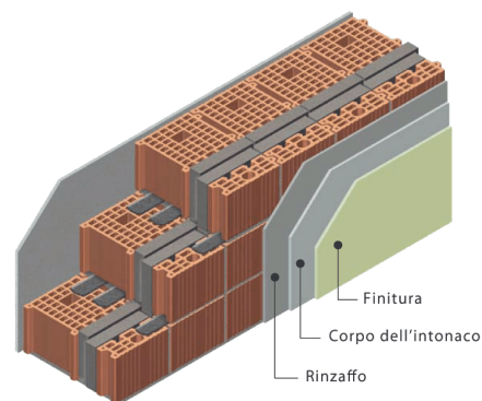
Gli strati dell'intonaco da https://t2d.it/prodotti-e-soluzioni/t2d-specialties/blocchi-con-isolante/tris-e-gli-intonaci/
