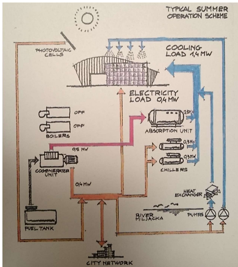
Fig. 3 - Concorso per l'auditorium di Sarajevo, schema del sistema di climatizzazione
