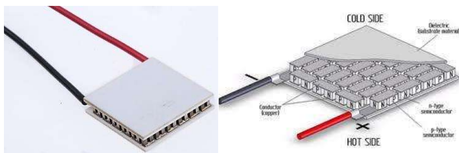
Fig. 15 – Cella di Peltier
