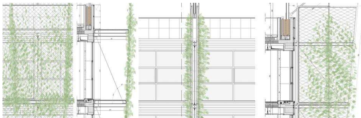
Fig. 5 - Prospetto e sezione del sistema tecnologico per facciata verde (schermo, sopra, e frangisole verticale, sotto)
