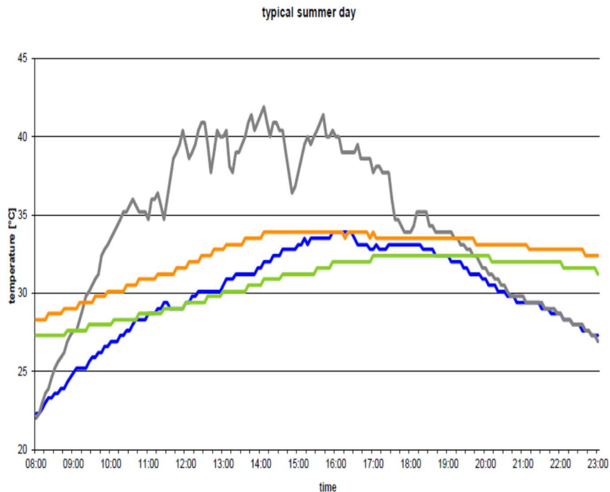
Fig. 17 – Confronto delle temperature interne dei due ambienti test (verde: facciata raffrescante; arancione: facciata ventilata), in rapporto all'irraggiamento solare (grigio) e alla temperatura esterna (blu) in una giornata estiva (Torino)
