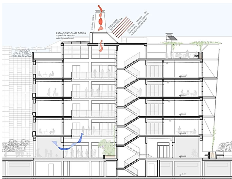
Fig. 6 - Edificio per uffici, sezione verticale, in evidenza l'effetto camino
