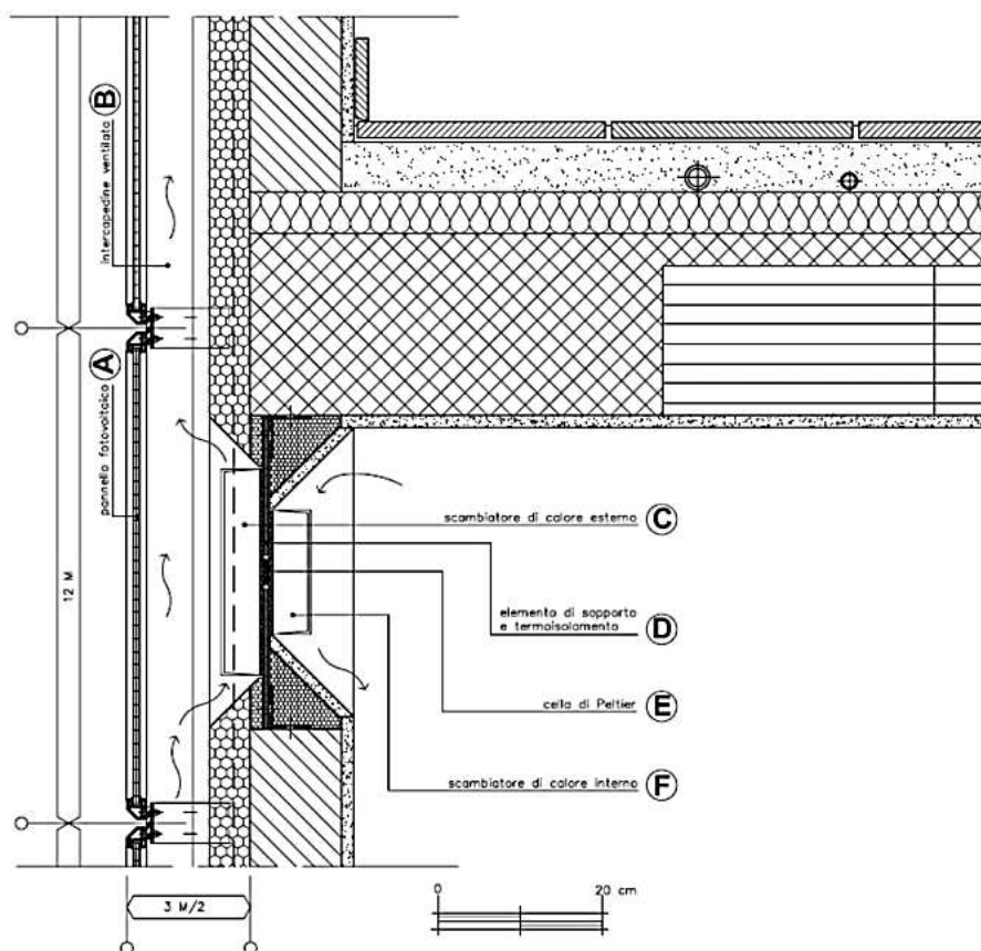
Fig. 16 – Sezione verticale del sistema di facciata raffrescante autoregolante
