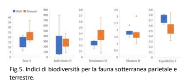
Fig. 5. Indici di biodiversità per la fauna sotterranea parietale e terrestre.
