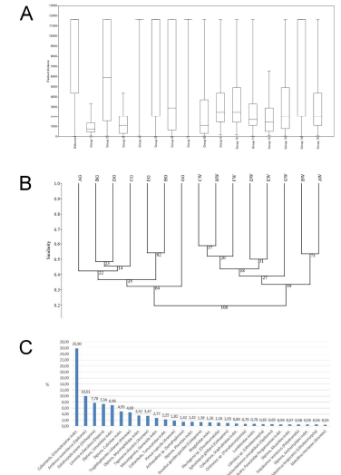
Fig. 4. A: One-way ANOSIM test. Pareti in otto siti (A-H, Gruppi 1-8), terreni in sette siti (A-E e G-H, Gruppi 9-15); B: somiglianza tra la fauna terrestre (da AG a HG) e quella parietale (da AW a HW) (clustering UPGMA basato su indice di somiglianza di Jaccard - i valori bootstrap sono mostrati sotto ogni nodo); C: Analisi SIMPER. Taxa responsabili delle differenze osservate tra le comunità nelle diverse aree di campionamento in percentuale.
