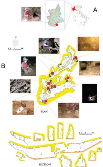
Fig. 1. A: Grotta del Baraccone, Piemonte, Italia (foto: E. Lana); B: Rilievo della grotta con le aree di monitoraggio. Quadrati rossi per il monitoraggio della fauna terrestre e triangoli blu per il monitoraggio della fauna parietale (mappa: V. Balestra e R. Sella, foto: E. Lana e V. Balestra).
