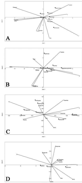
Fig. 3. Canonical Correspondence Analysis. Fauna ipogea legata a fattori ambientali e substrato minerale. A: Classi di fauna terrestre; B: Ordini di fauna terrestre (Arachnida, Entognatha e Insecta) con un numero di esemplari superiore al 5% del totale di ciascuna classe considerata; C: Classi di fauna parietale; D: Ordini di fauna parietale (Arachnida e Insecta) con un numero di esemplari superiore al 5% del totale di ciascuna classe considerata.
