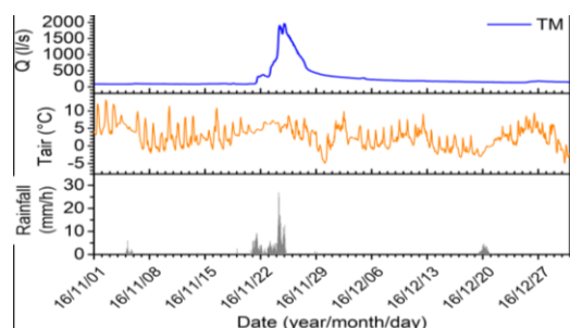
Fig. 22 – Andamento della portata del collettore in seguito all'evento alluvionale del novembre 2016
