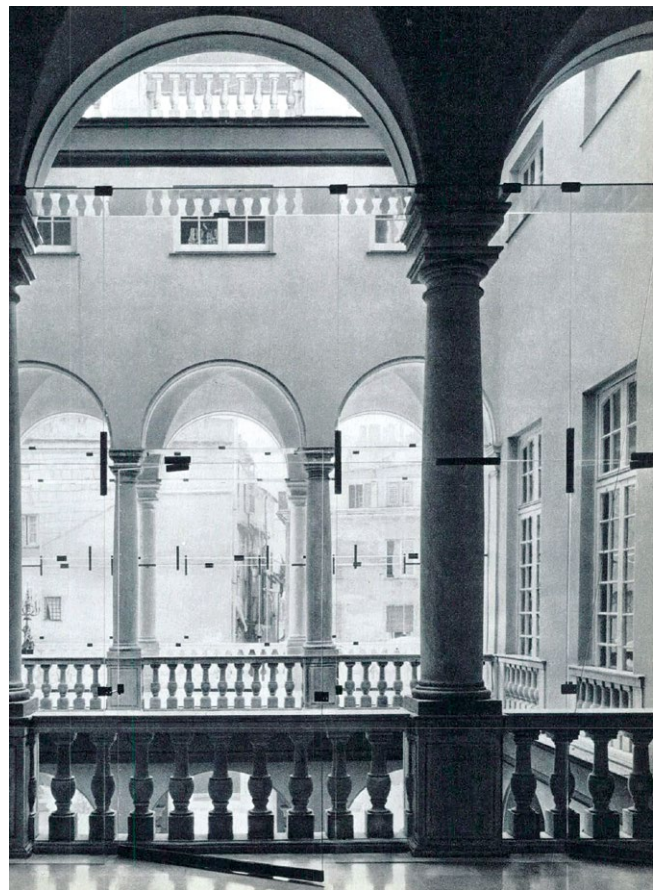
fig. 6 – Dettaglio delle chiusure verticali scelte da Albini per il loggiato di Palazzo Rosso, 1963 (da «Domus», n. 408, p. 43).
