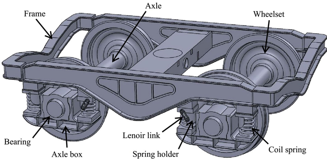
Fig. 3 Y25 bogie
