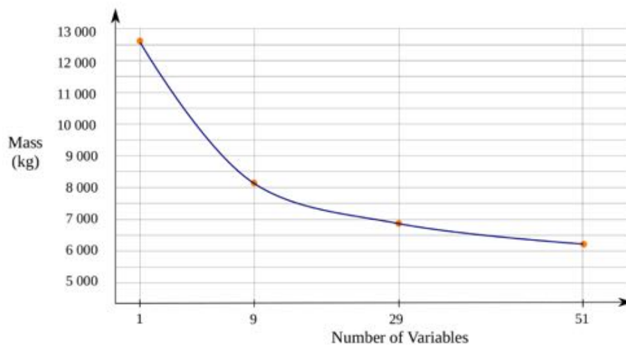
Fig. 7. Pareto front
