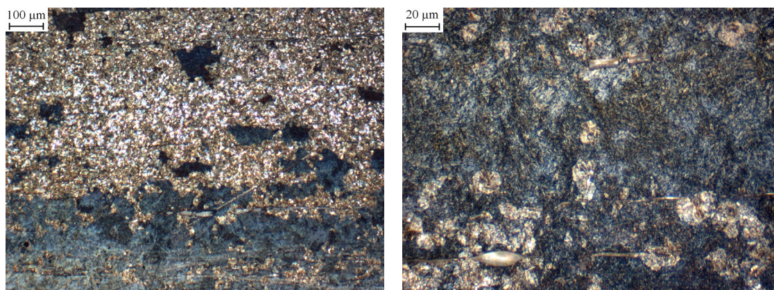
Fig.9 - Microstrutture nella lama della spada II (campione II-L2, sezione longitudinale, microscopia ottica): microstruttura a bande (a), martensite e perlite fine nella regione ad alto tenore di carbonio in prossimità della superficie (b). - Microstructures in the blade of sword II (sample II-L2, longitudinal section, light microscopy): banded microstructure (a), martensite and fine perlite in the high-carbon region near the surface (b).
