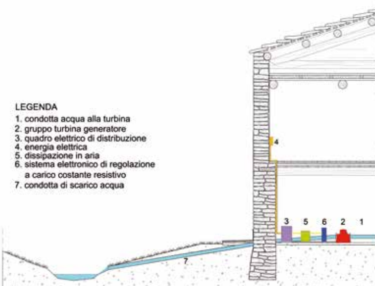
Schema di impianto microidroelettrico.
