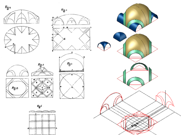
Figure 2. Banded vault in the Architettura civile by Guarini. Source: Guarini, 1737. Modeling: R. Spallone
