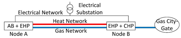
Fig. 14. Test system 3.
