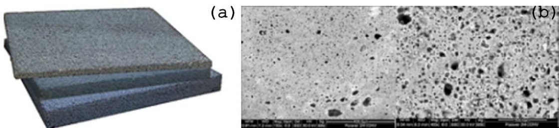
Figura 1 – Pannelli 54 \times 54 \text{ cm} di diversi spessori, A= 16 \pm 1 \text{ mm} , B= 37 \pm 2 \text{ mm} , C= 57 \pm 3 \text{ mm} (a) e immagine SEM dell'aggregato sezionato (b) – 54 \times 54 \text{ cm} Panels of three thicknesses, A= 16 \pm 1 \text{ mm} , B= 37 \pm 2 \text{ mm} , C= 57 \pm 3 \text{ mm} (a) and SEM image of the aggregate section (b).
