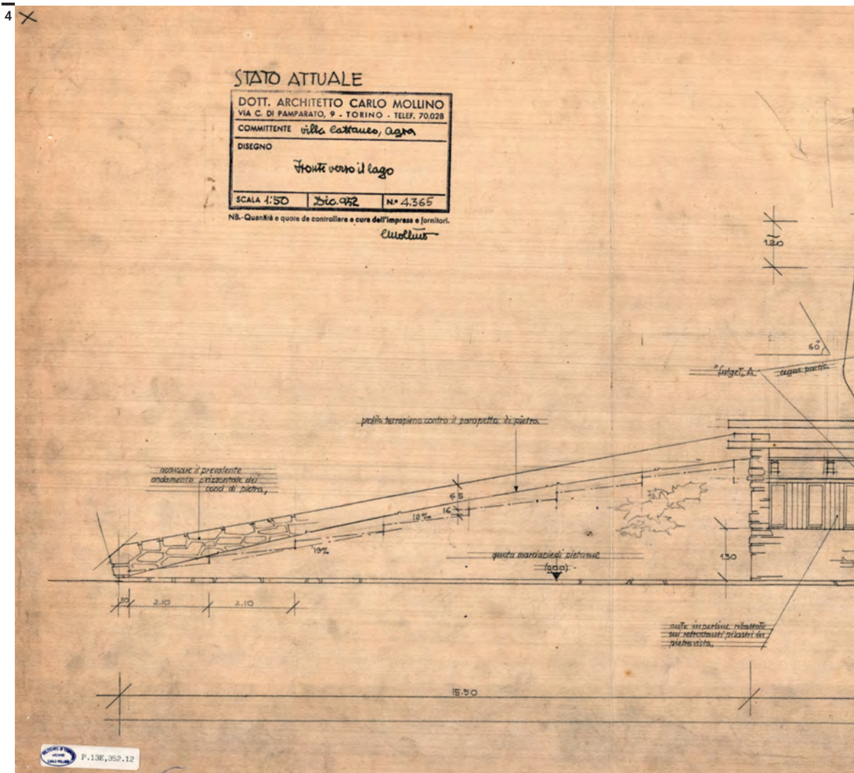
Fig. 4 Tavole di progetto, prospetto del fronte verso il lago.
