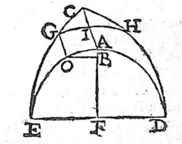
Fig. 3. Lunetta a tutto sesto e porzioni di essa. Immagine: Guarini 1674, Prop. 14; modellazione digitale: Roberta Spallone.
