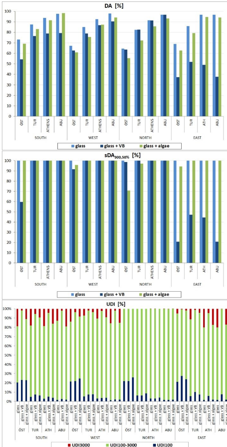
Fig. 13. Parametric study: DA, sDA 300/50% and UDI values.
