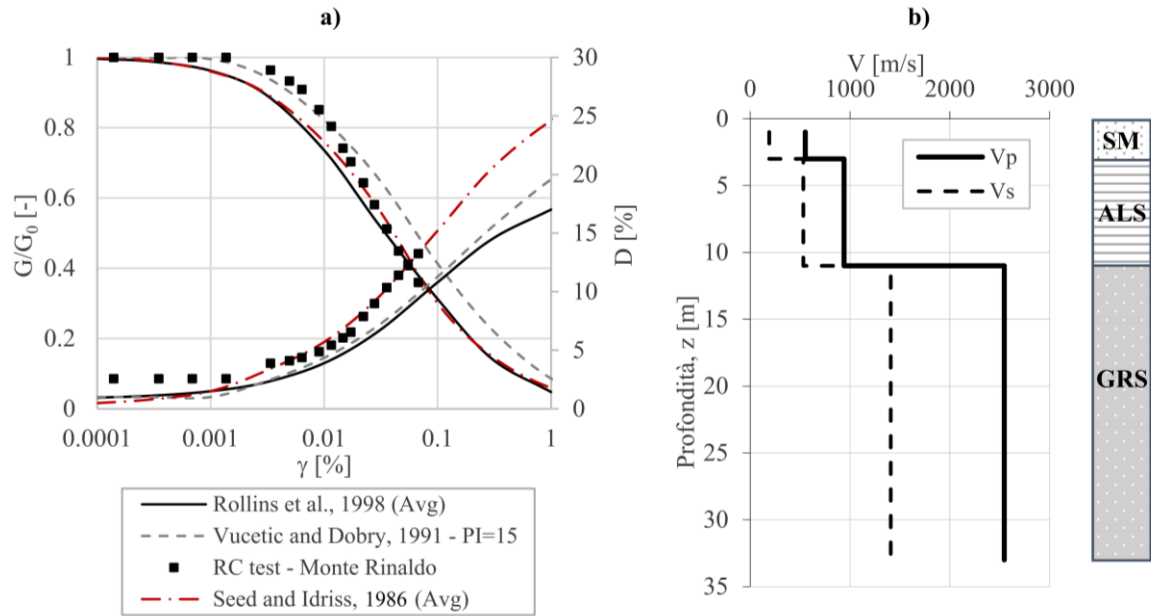
Figura 2: Modello di sottosuolo: a) curve di variazione del modulo di rigidità a taglio e del rapporto di smorzamento; b) profilo di V_s e V_p ottenuto mediante DHT.
